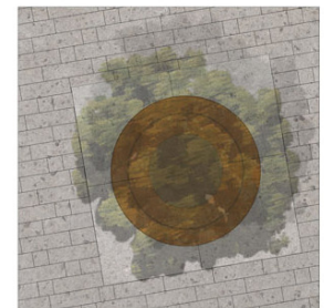
4. részlet M=1:25
