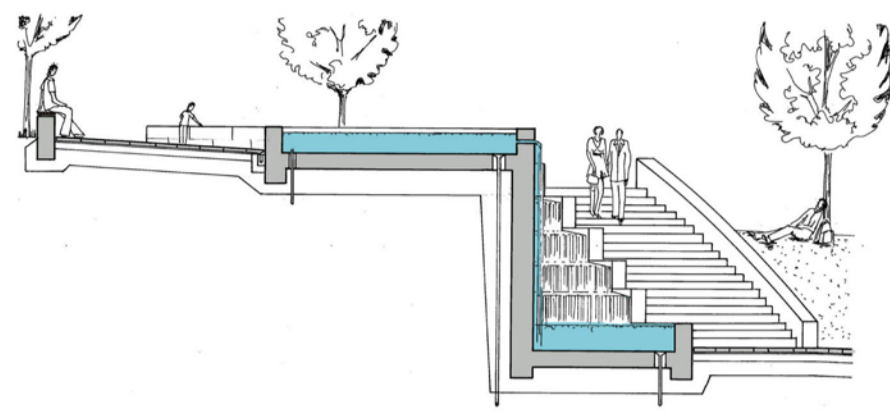
Vízésés metszet M=1:100
