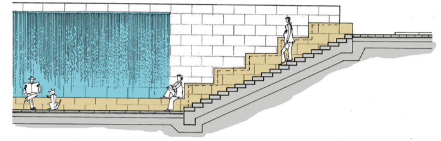
Kaszkád – lépcső metszet M= 1:100
