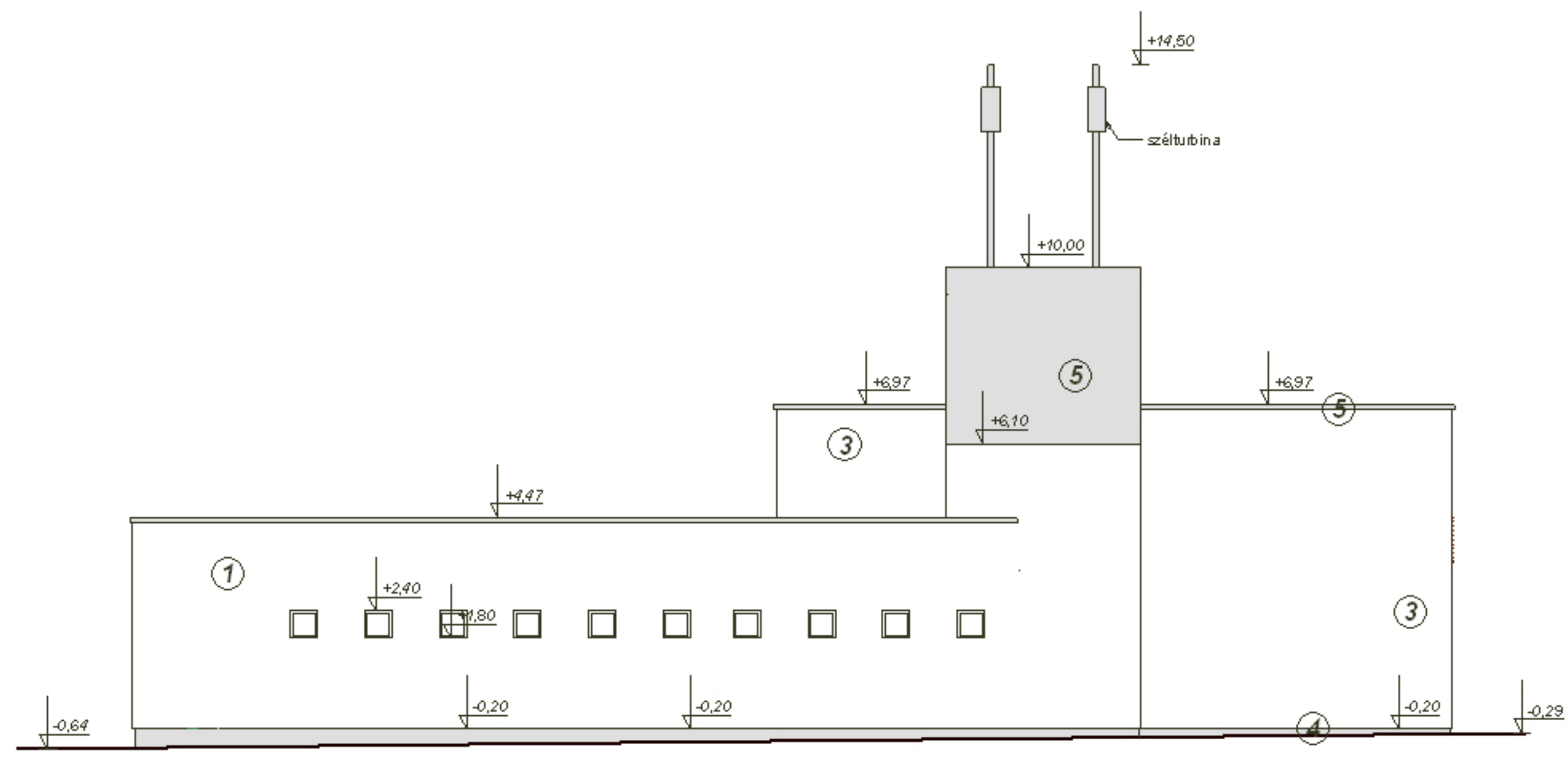
ÉSZAKI HOMLOKZAT
