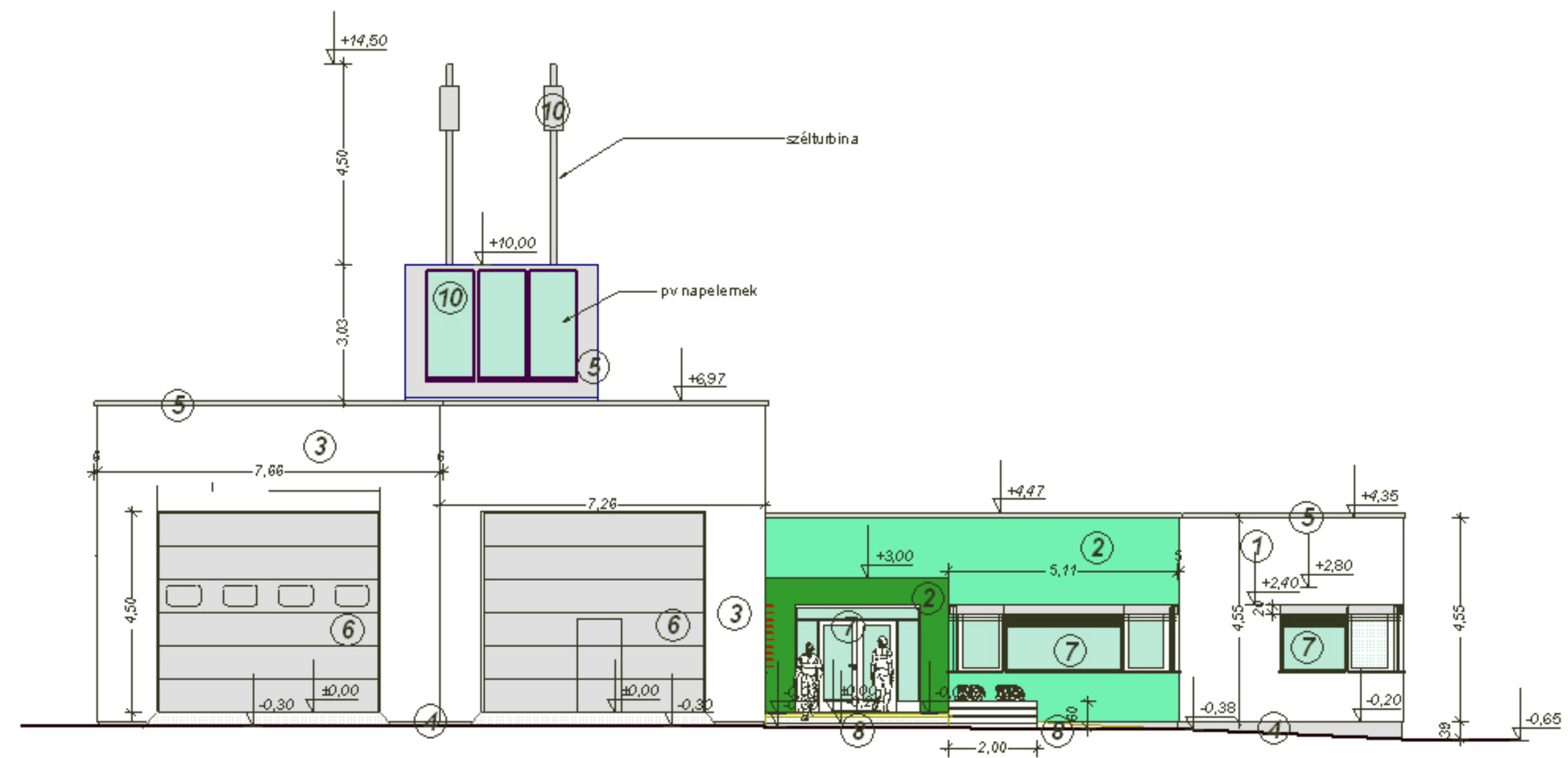
DÉLI HOMLOKZAT
