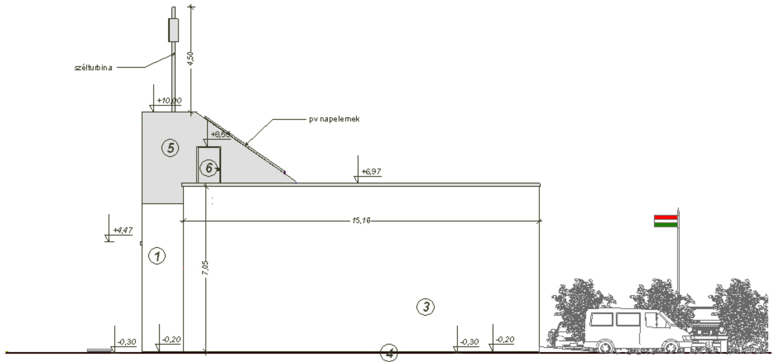
KELETI HOMLOKZAT
