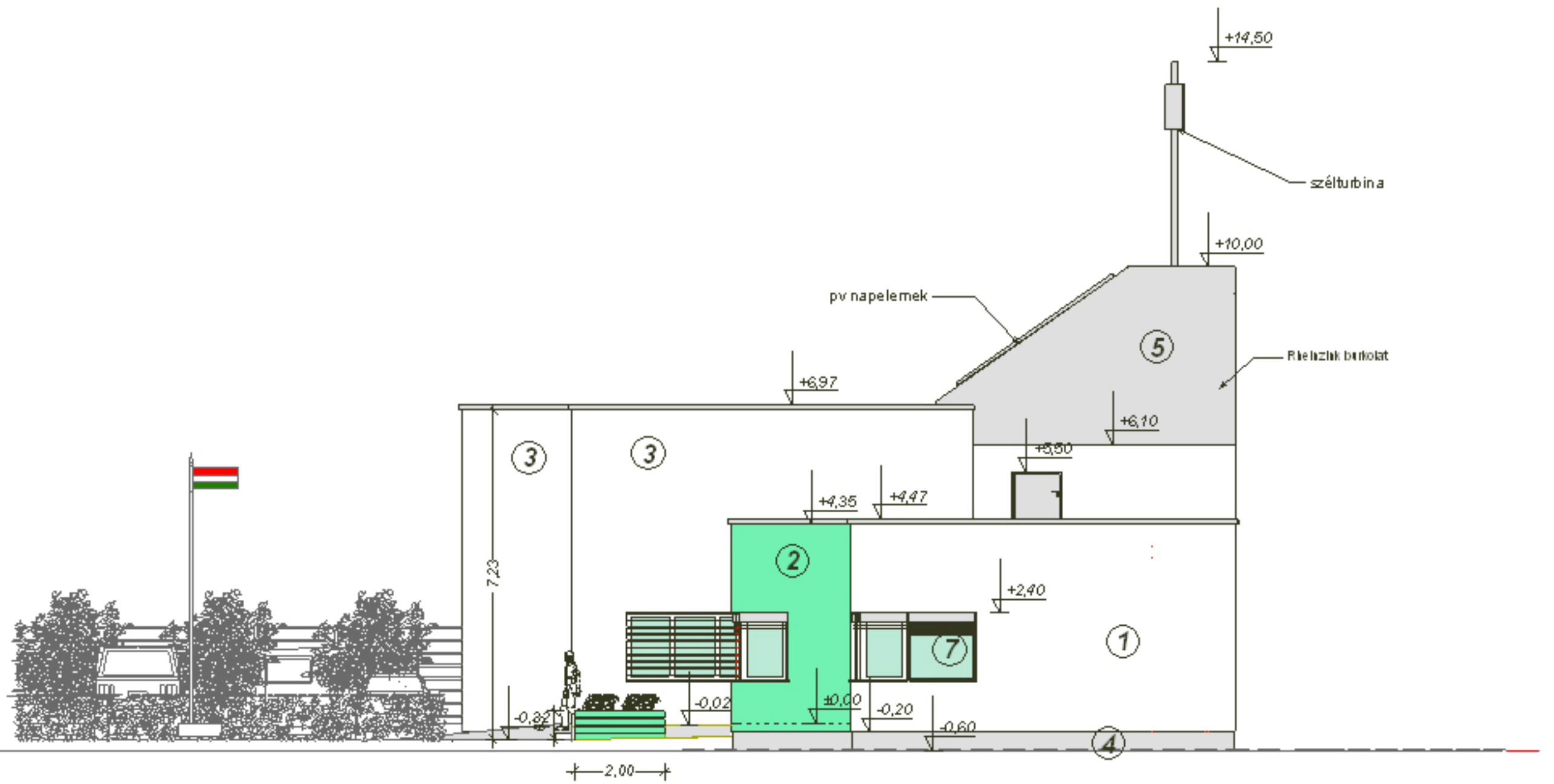
KELETI HOMLOKZAT
