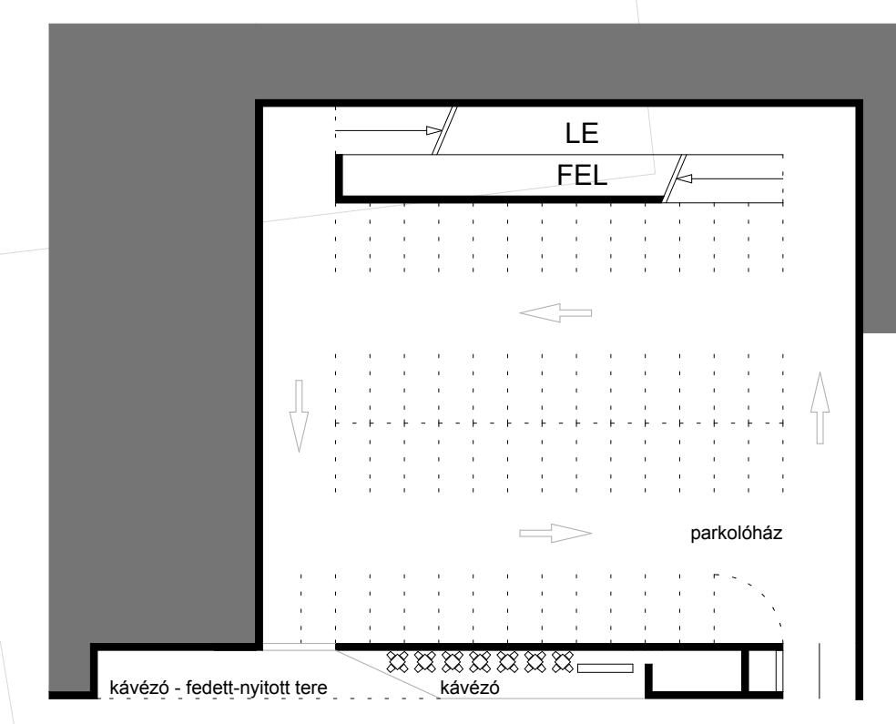
PARKOLÓHÁZ FÖLDSZINTI ALAPRAJZ M = 1 : 500
