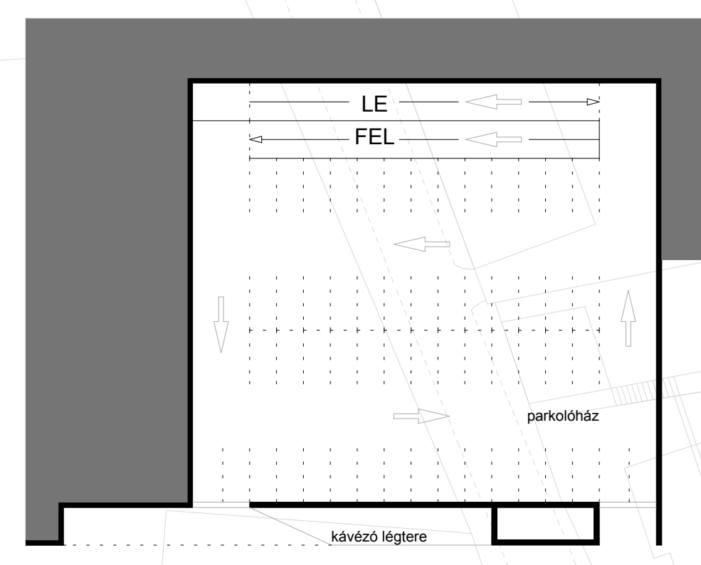
PARKOLÓHÁZ EMELETI ALAPRAJZ M = 1 : 500
