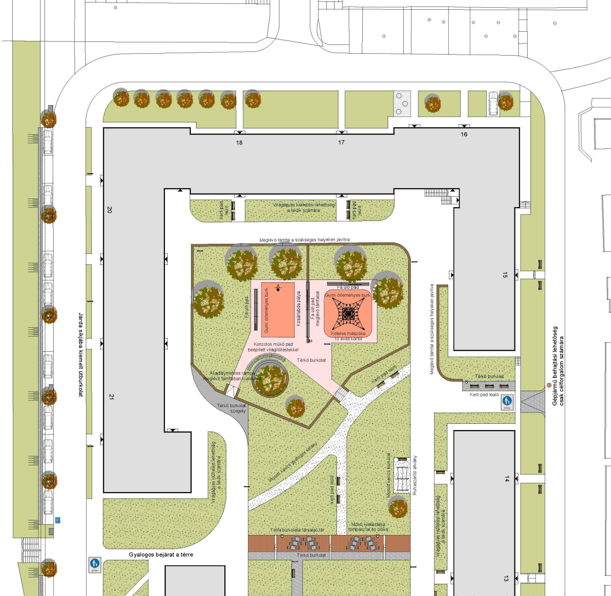
FEKETEGYÉMÁNT TÉR RÉSZLET M 1:200
