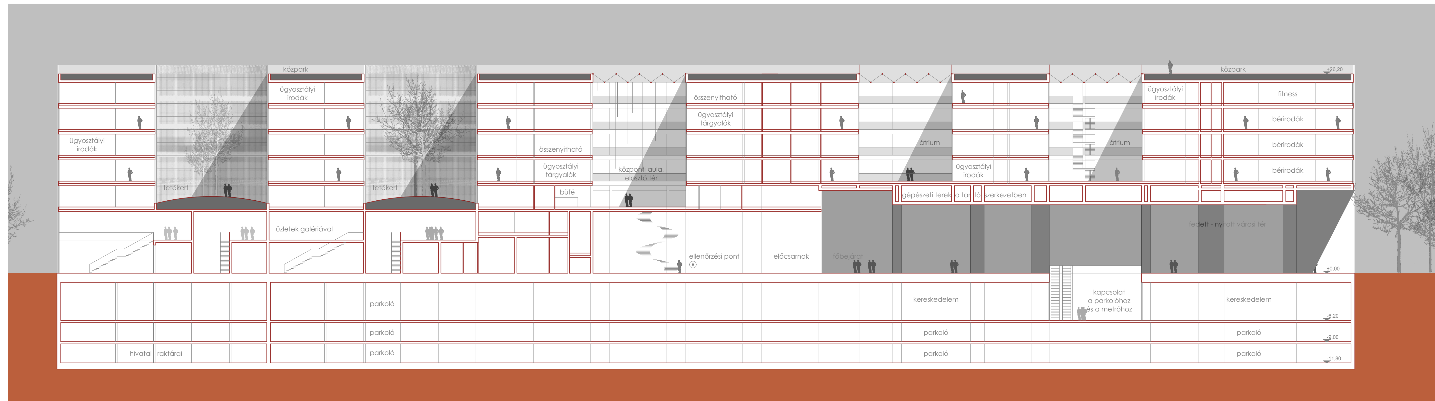
C - C METSZET 1:250
