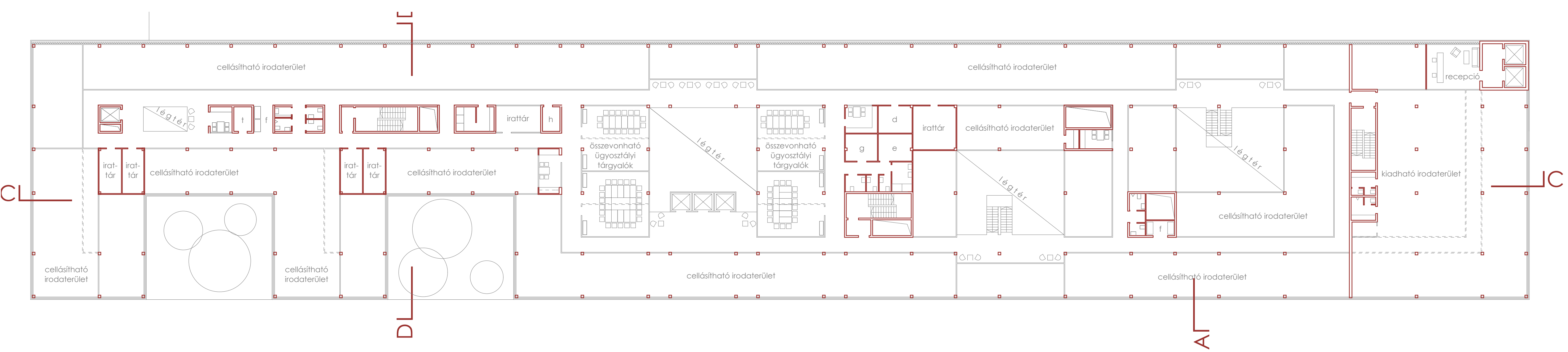
3. EMELET ALAPRAJZ 1:250
