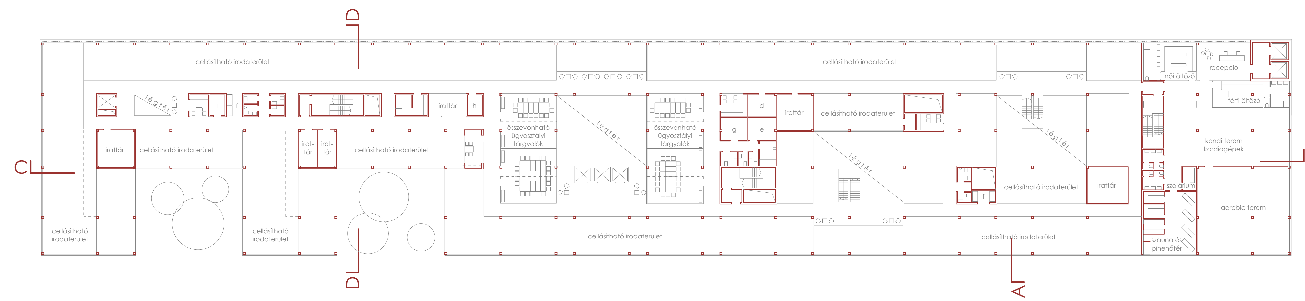
5. EMELETI ALAPRAJZ 1:250
