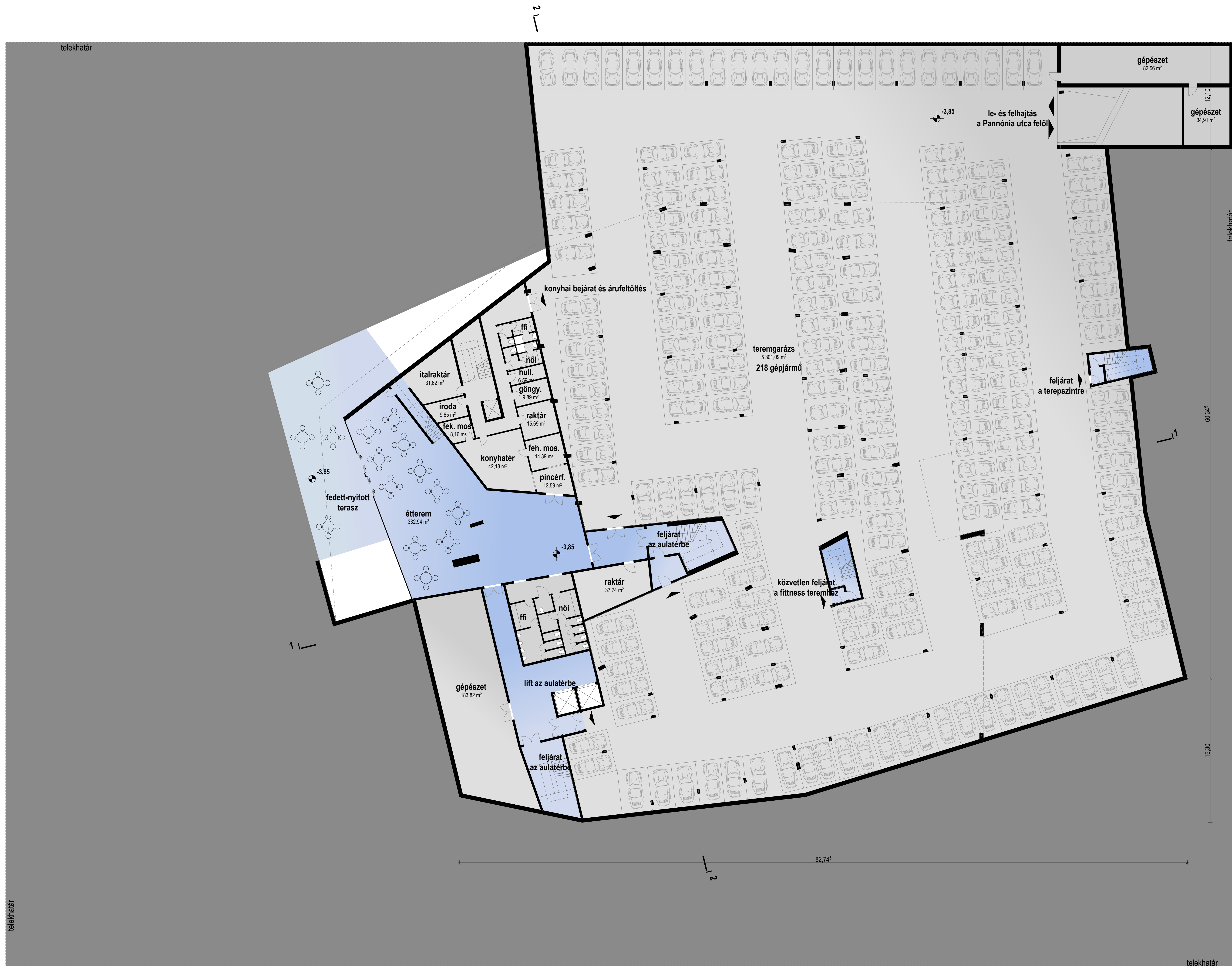
PINCE ALAPRAJZ - M 1:200
