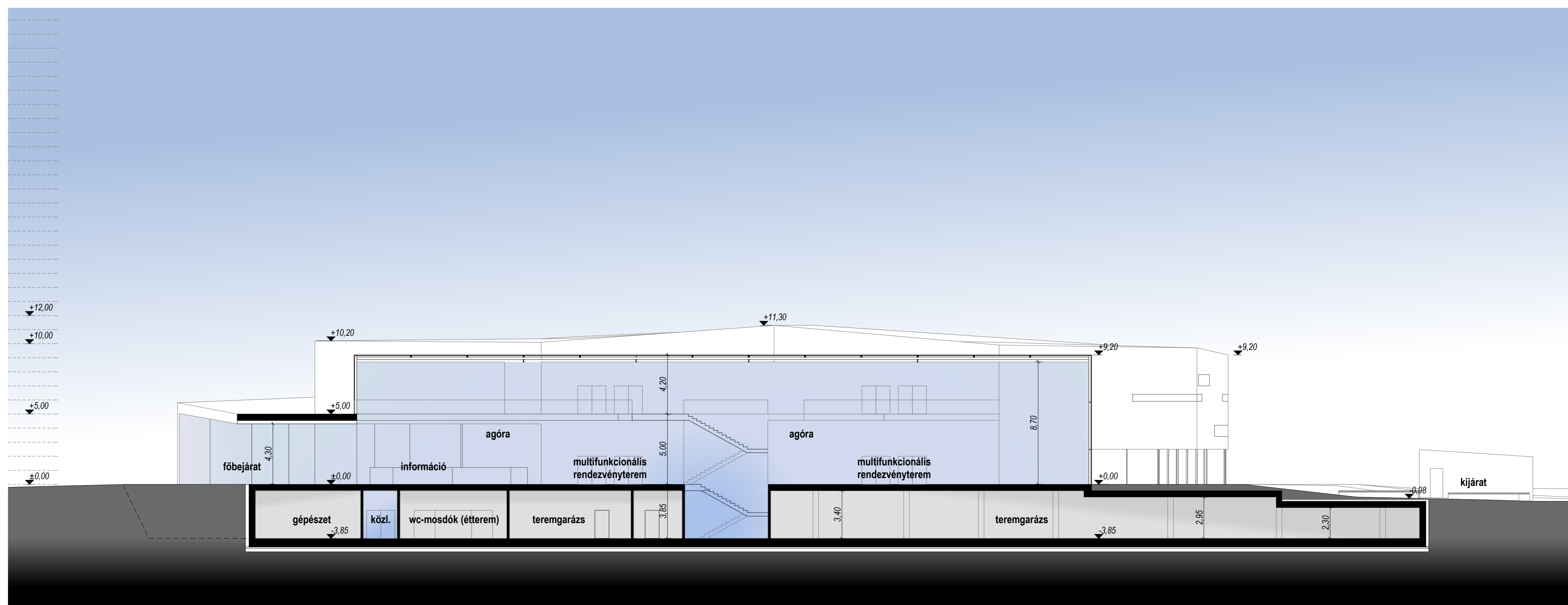
1-1 metszet - M 1:200
