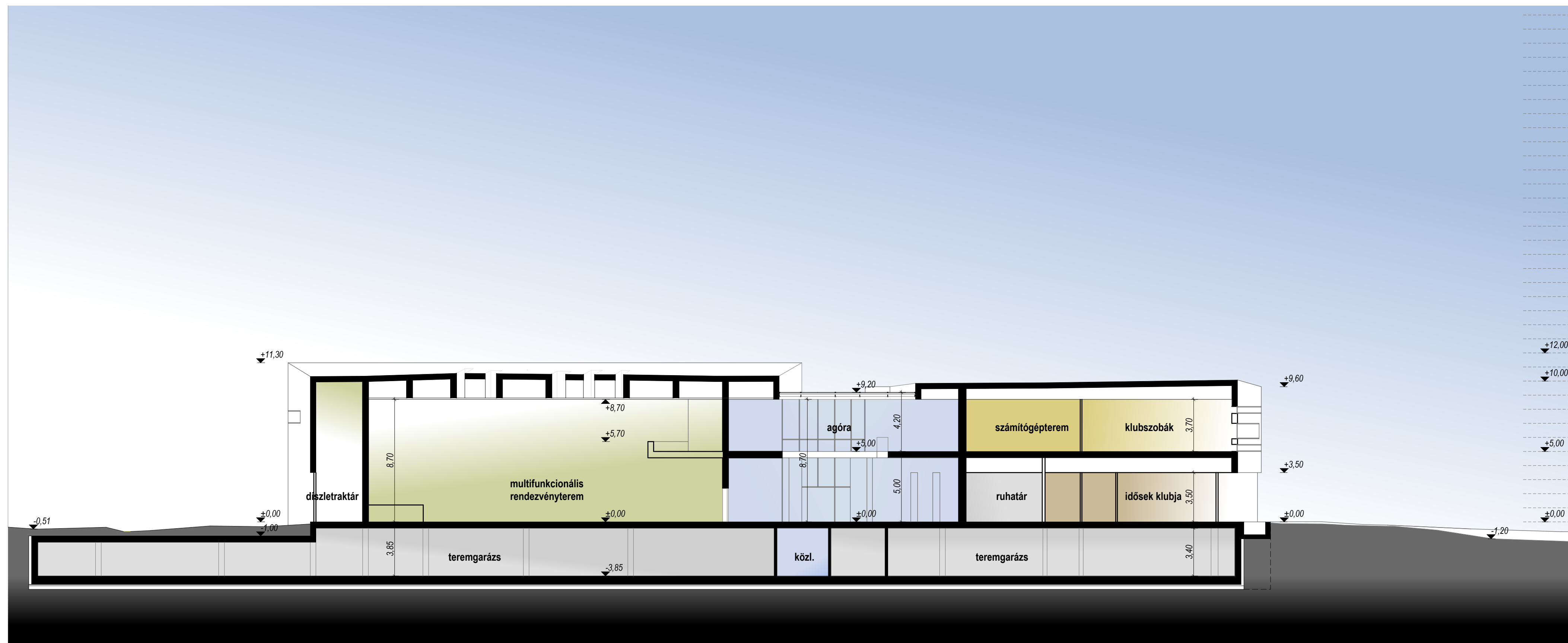
2-2 metszet - M 1:200
