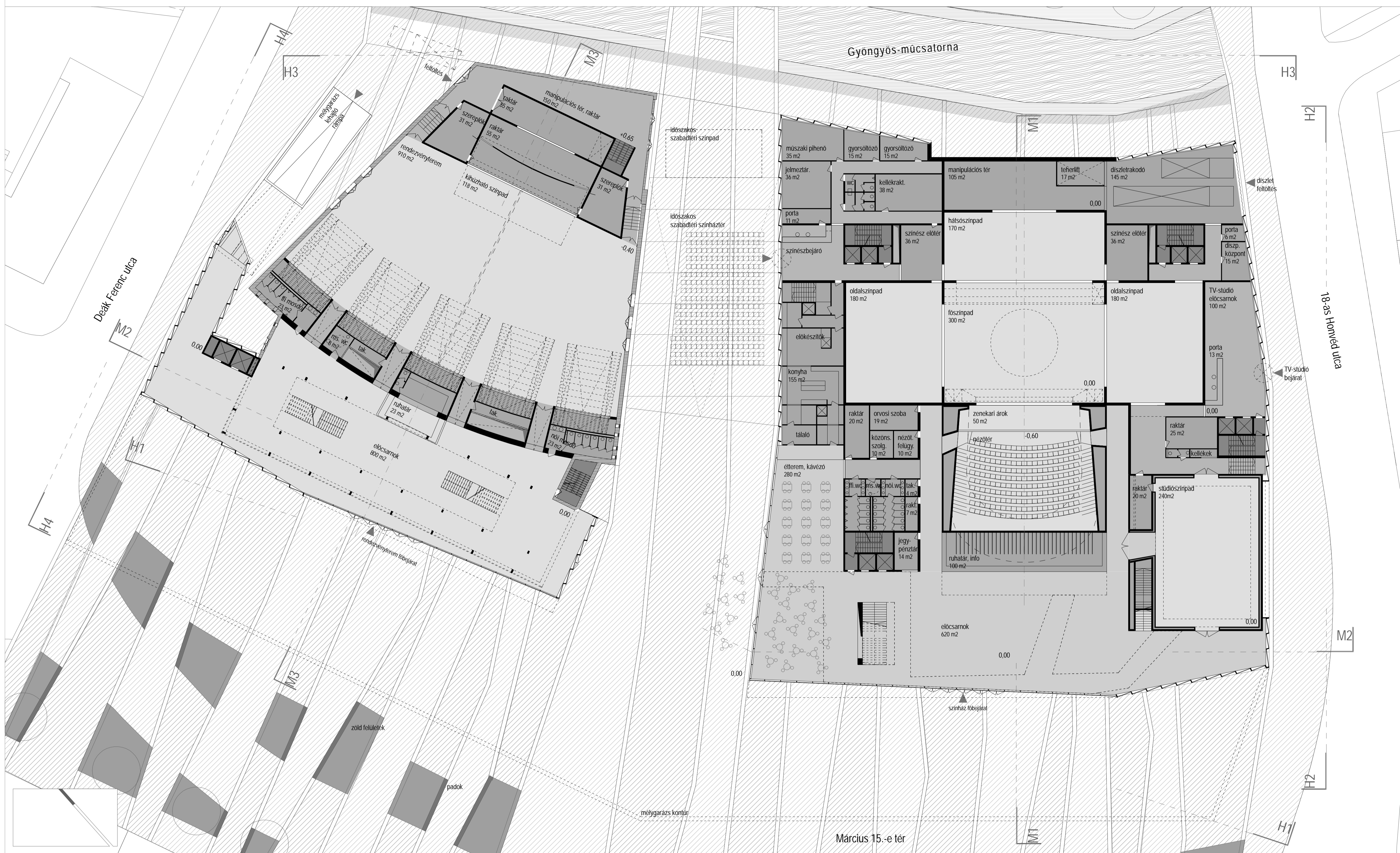
FÖLDSZINTI ALAPRAJZ
