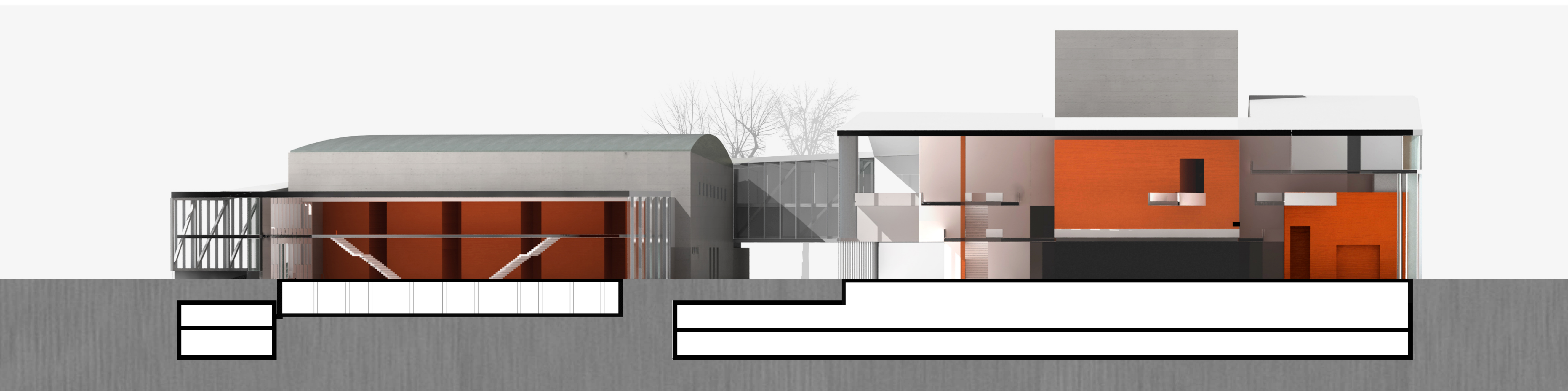
M-2 METSZET M 1:250
