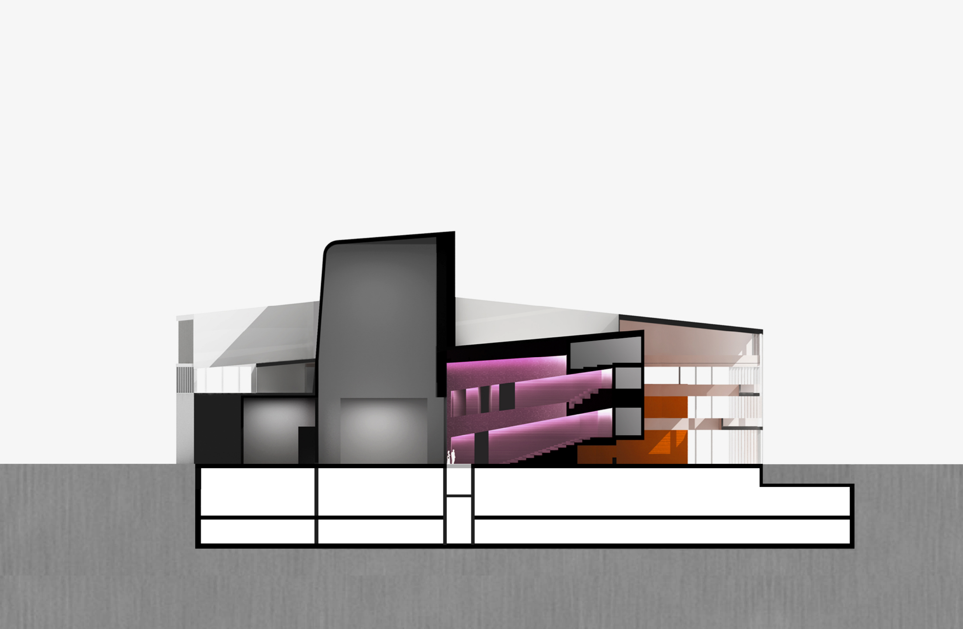
M-1 METSZET M 1:250
