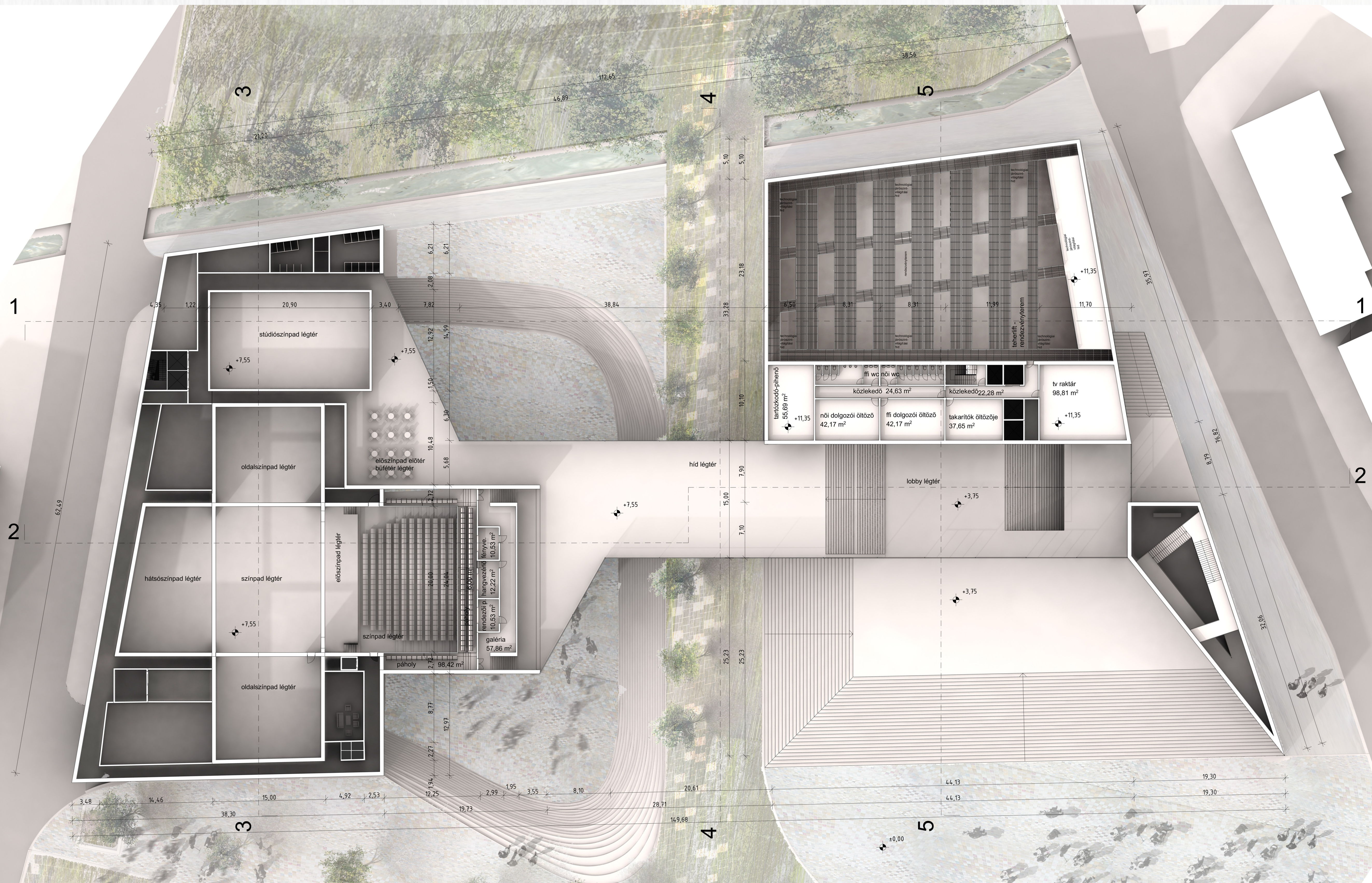
TECHNIKAI ÉS PÁHOLY SZINT ALAPRAJZ M 1:250
