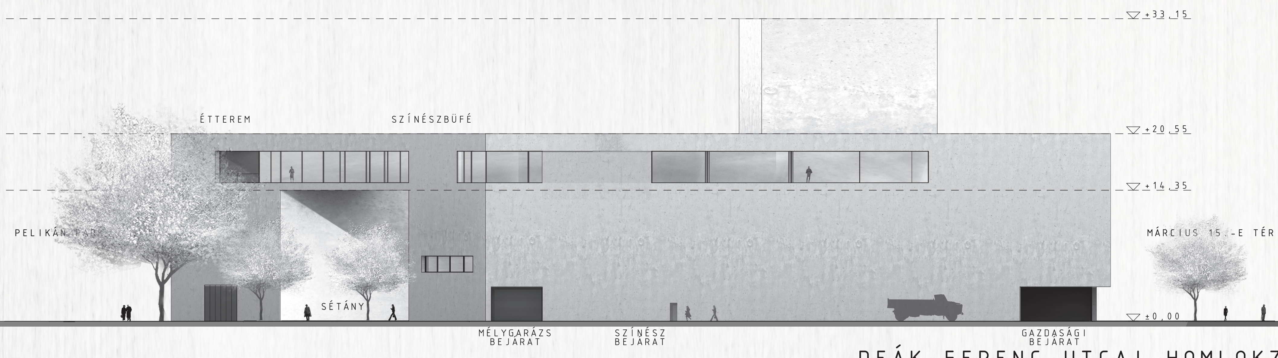
DEÁK FERENC UTCAI HOMLOKZAT M1:250
