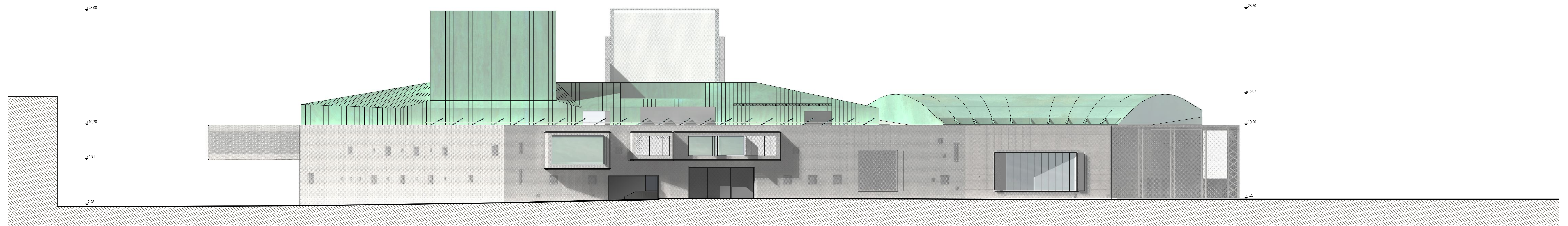
KELETI HOMLOKZAT M 1:250
