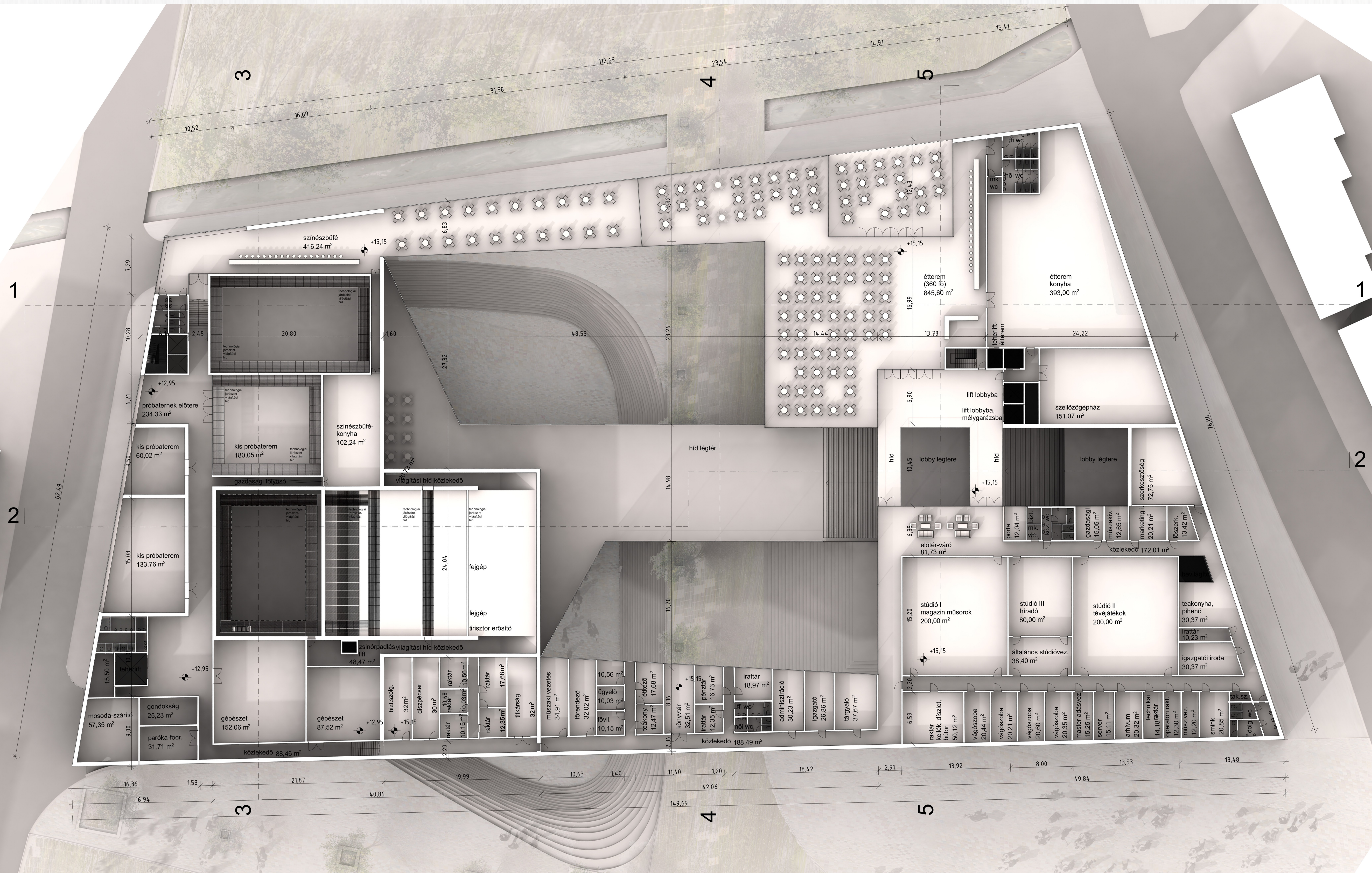
TV, ÉTTEREM, PRÓBATEREM, IRODA ALAPRAJZ M 1:250
