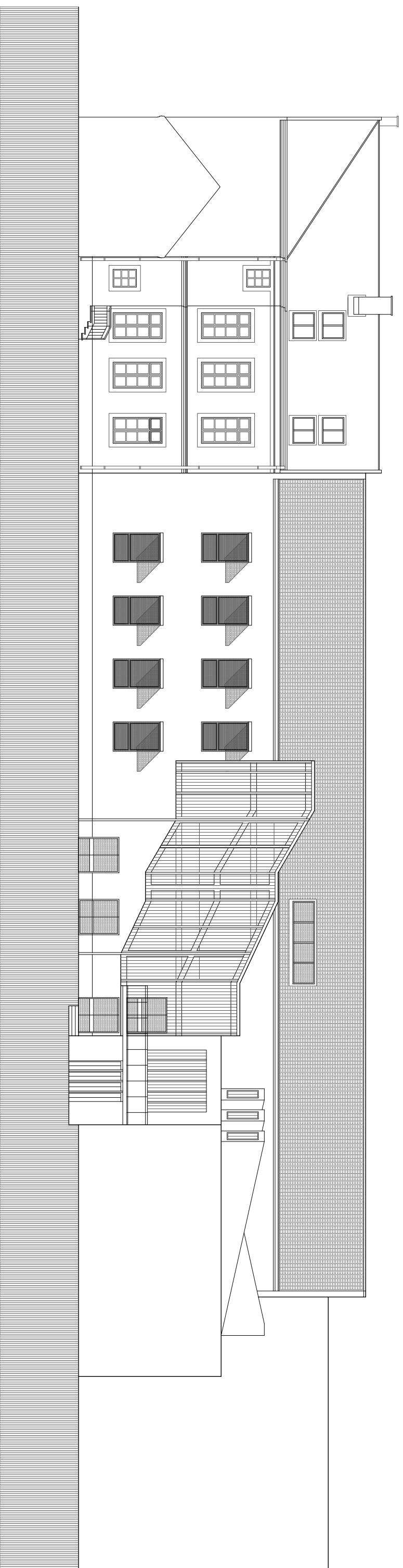
Belső udvar felőli homlokzat 1:200
