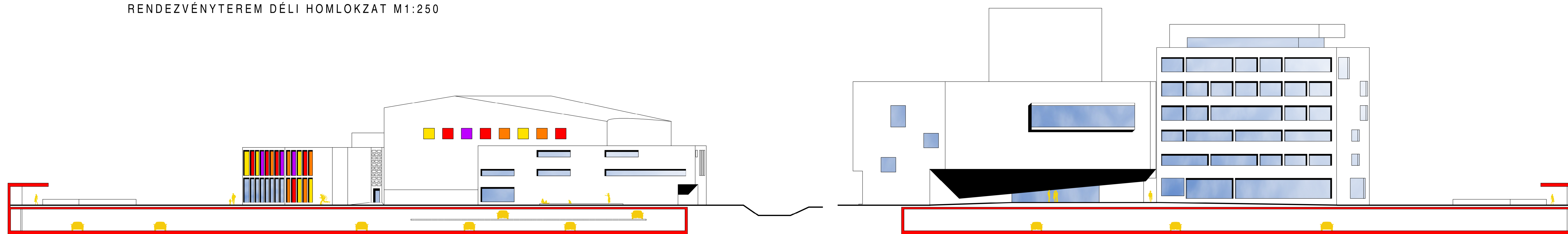
RENDEZVÉNYTEREM DÉLI HOMLOKZAT M1:250
