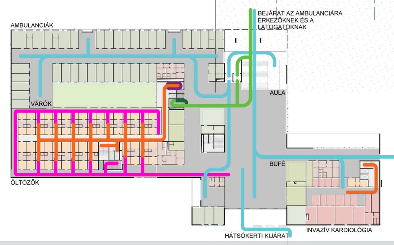
ÚTVONAL DIAGRAM M1:750
