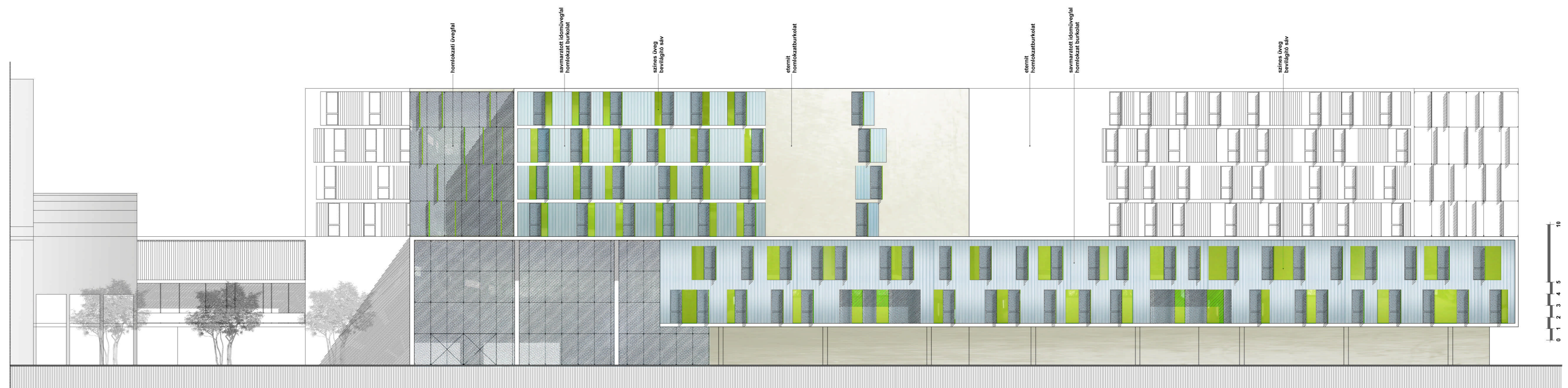
NYUGATI HOMLOKZAT M1:200
