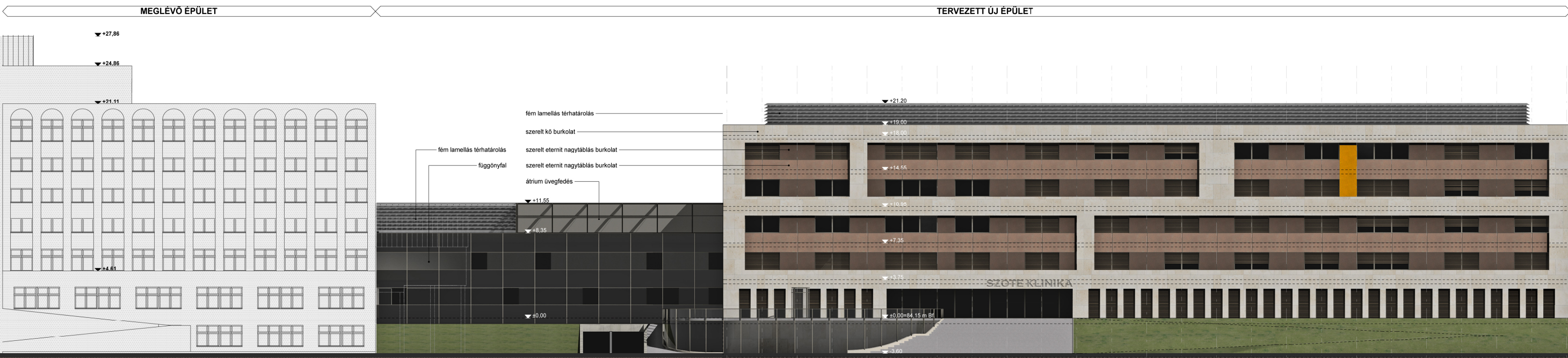
NYUGATI - SEMMELWEIS UTCAI HOMLOKZAT
