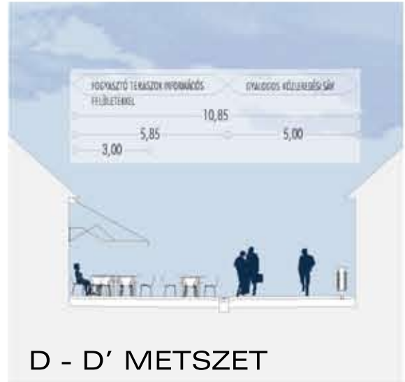
D - D' METSZET
