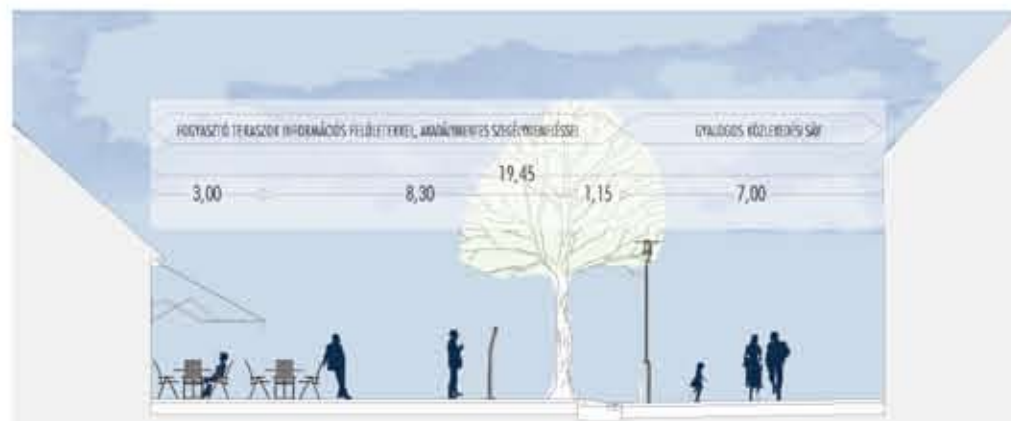
J - J' METSZET
