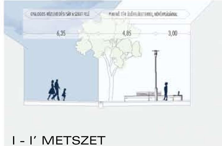
I - I' METSZET
