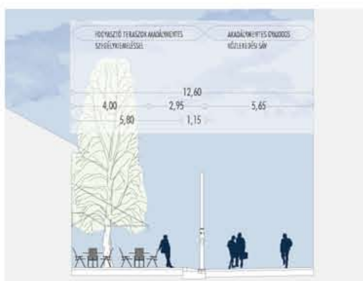
B - B' METSZET
