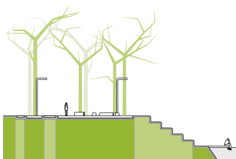
metszet általános helyen
