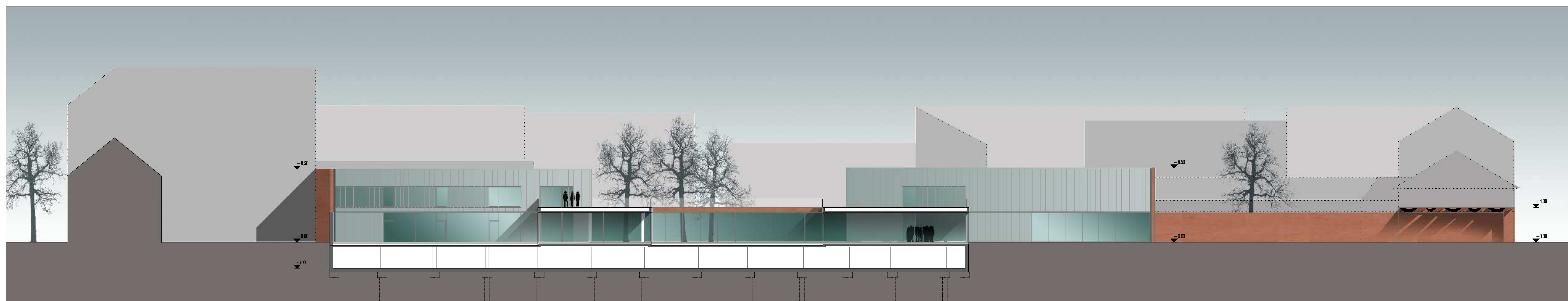
C-C METSZET
