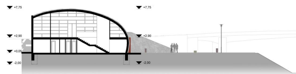
METSZET M 1:200
