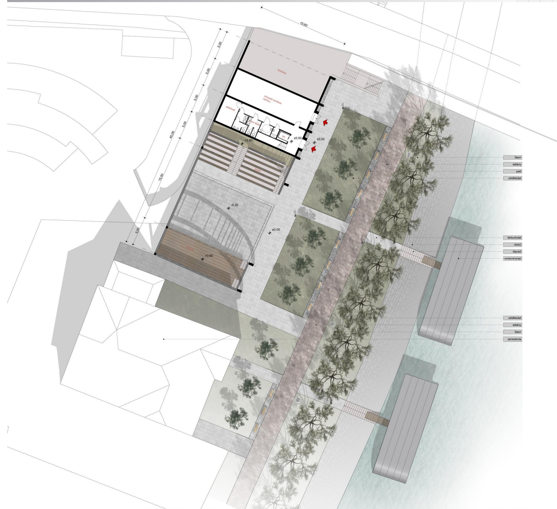
Fogadóépület és Színpad - FÖLDSZINTI ALAPRAJZ M 1:200
