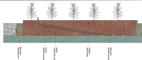
Stég NÉZET ALACSONY VIZÁLLÁSNÁL M 1:200
