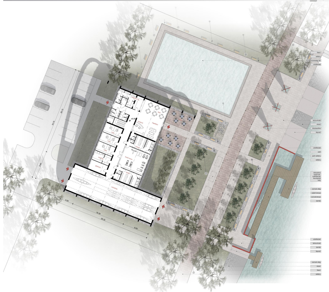
Csónakház - Földszinti Alaprajz M 1:200
