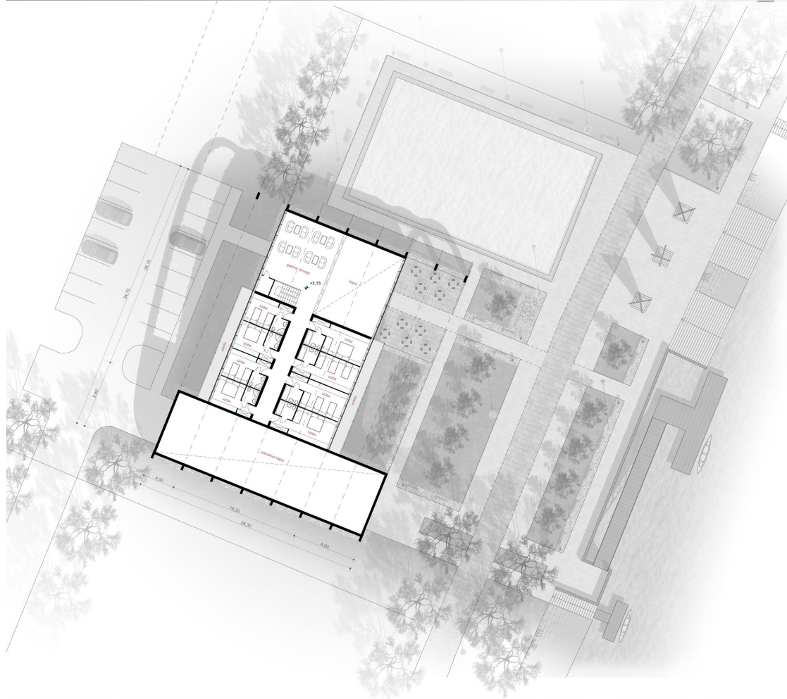
Csónakház - EMELETI ALAPRAJZ M 1:200
