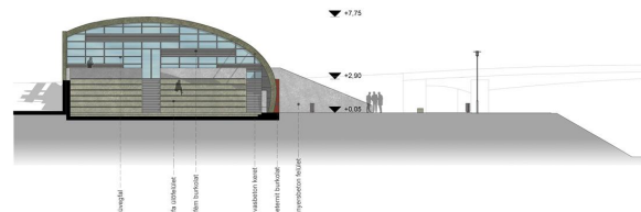
HOMLOKZAT M 1:200
