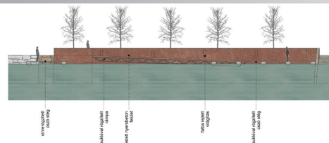
Stég NÉZET MAGAS VIZÁLLÁSNÁL M 1:200
