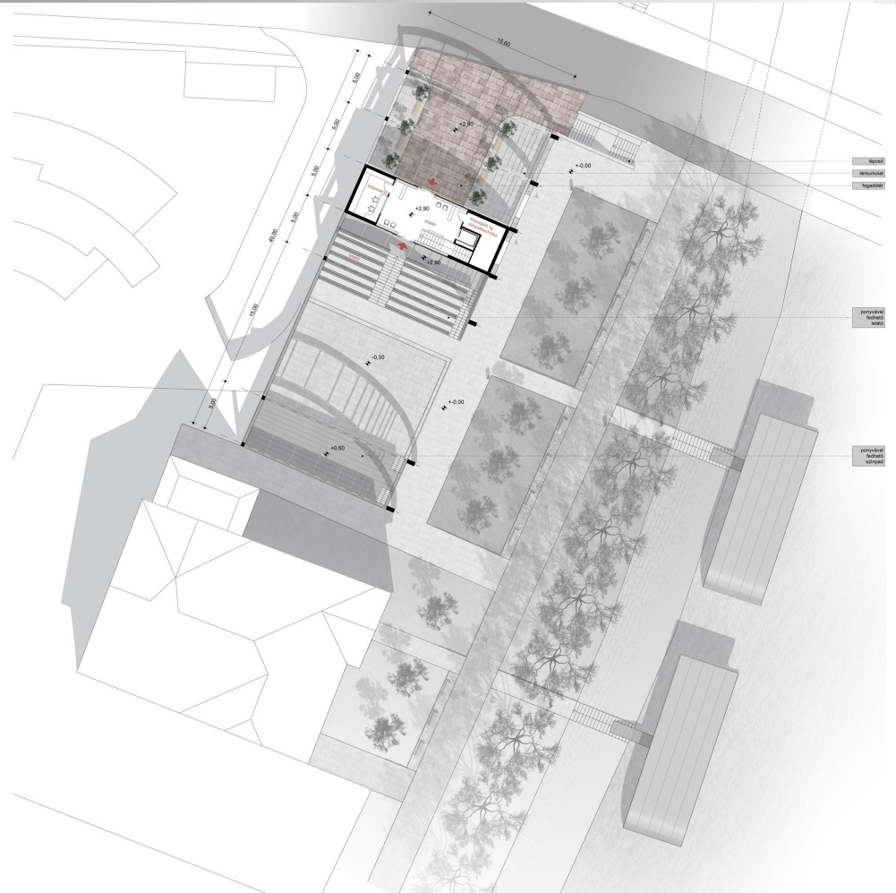
FOGADÓÉPÜLET ÉS SZÍNPAD - ÉMELETI ALAPRAJZ M 1:200
