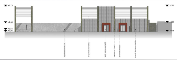
HOMLOKZAT M 1:200
