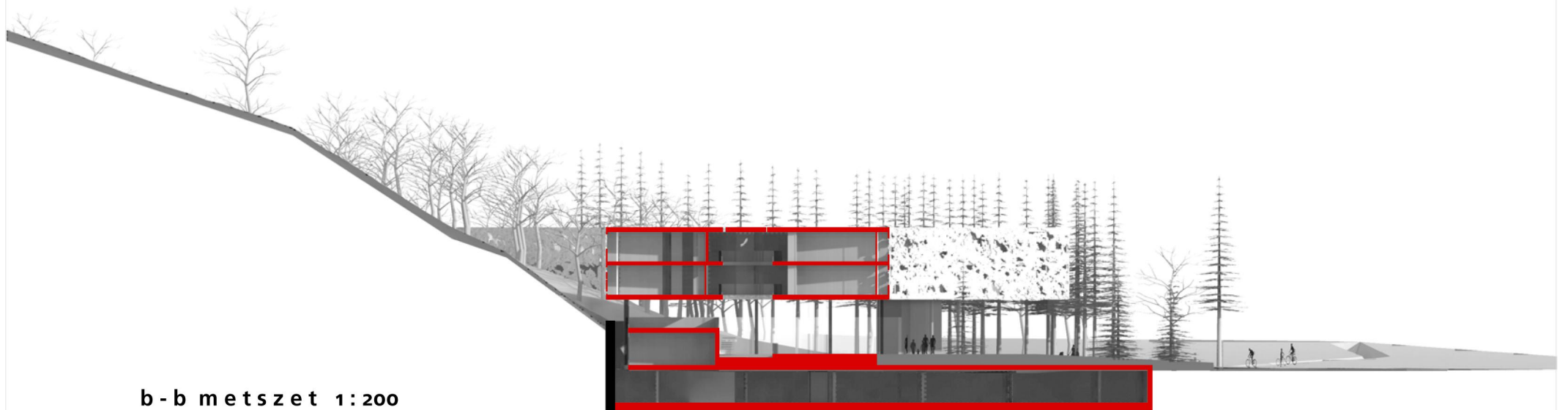
a-a metszet 1:200
