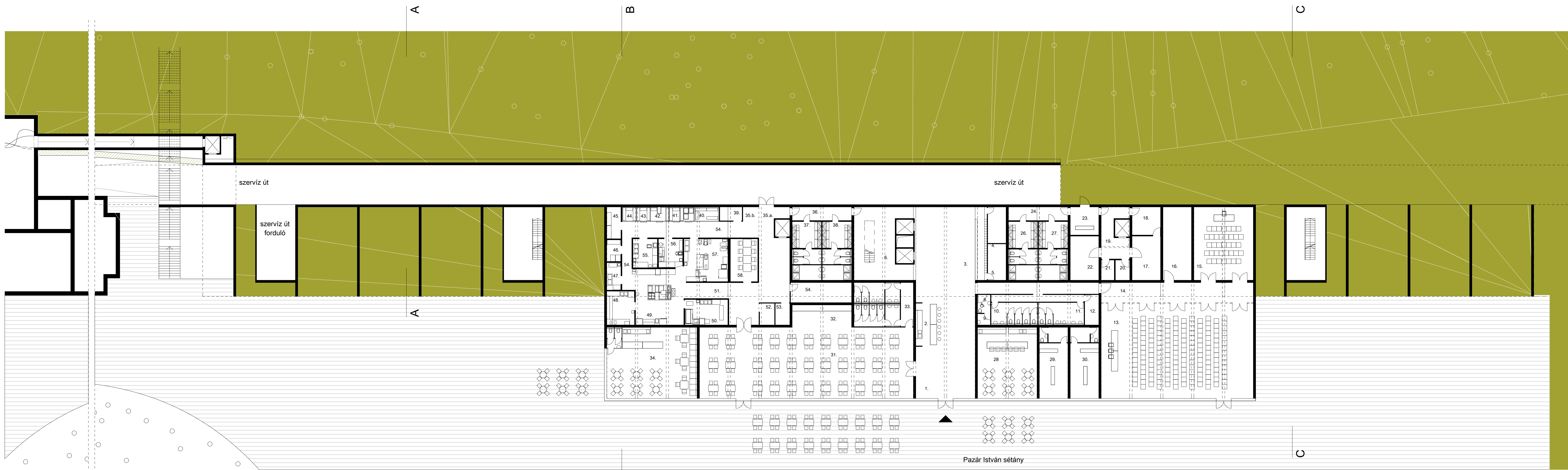
FÖLDSZINTI ALAPRAJZ
