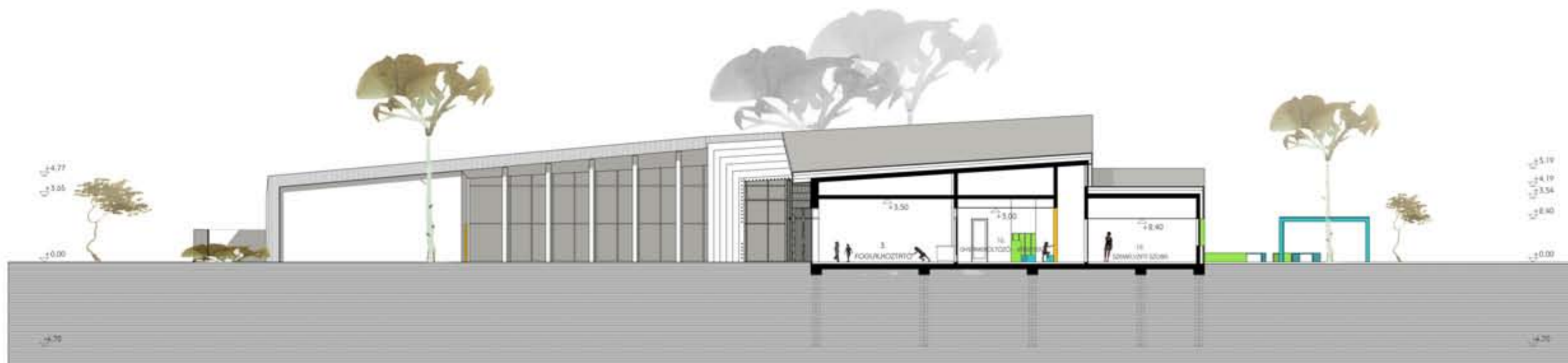
B-B METSZET
