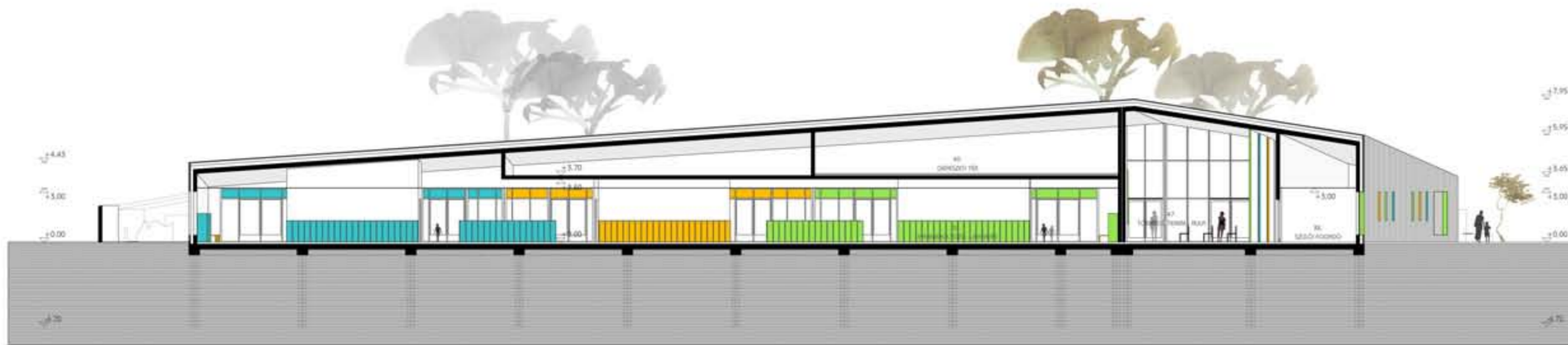
A-A METSZET
