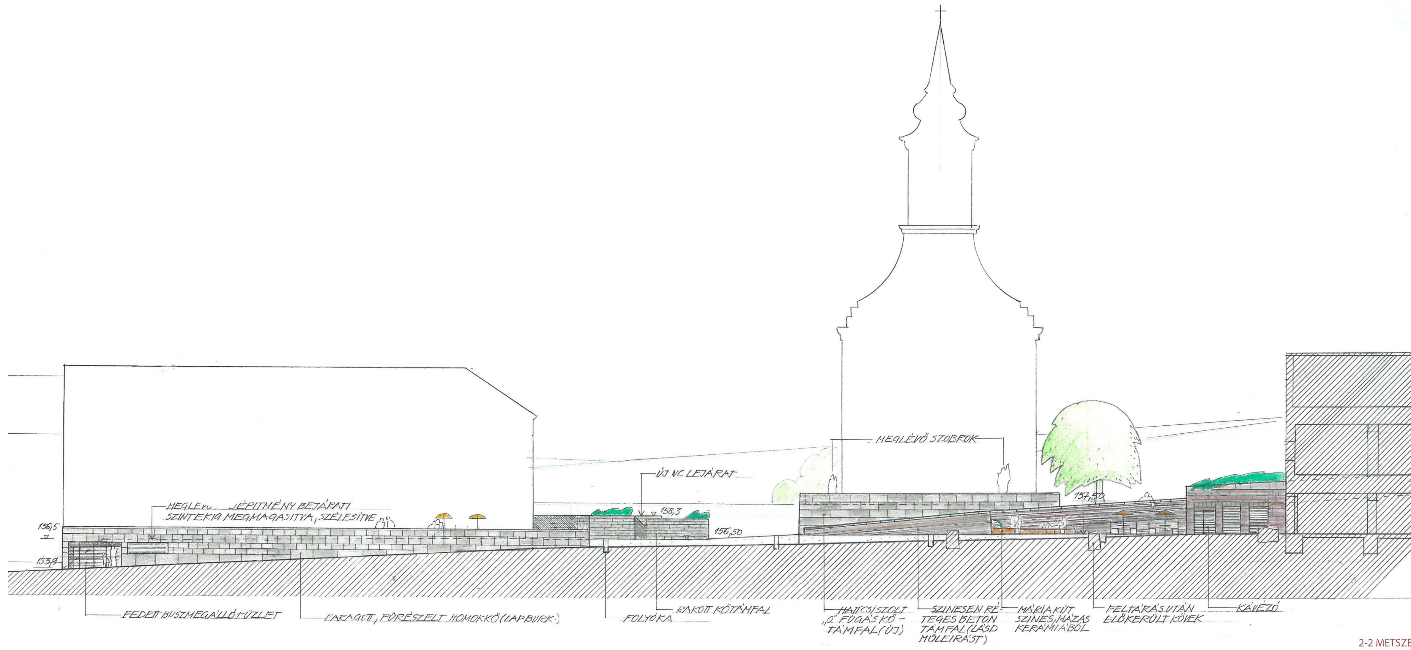
2-2 METSZET
