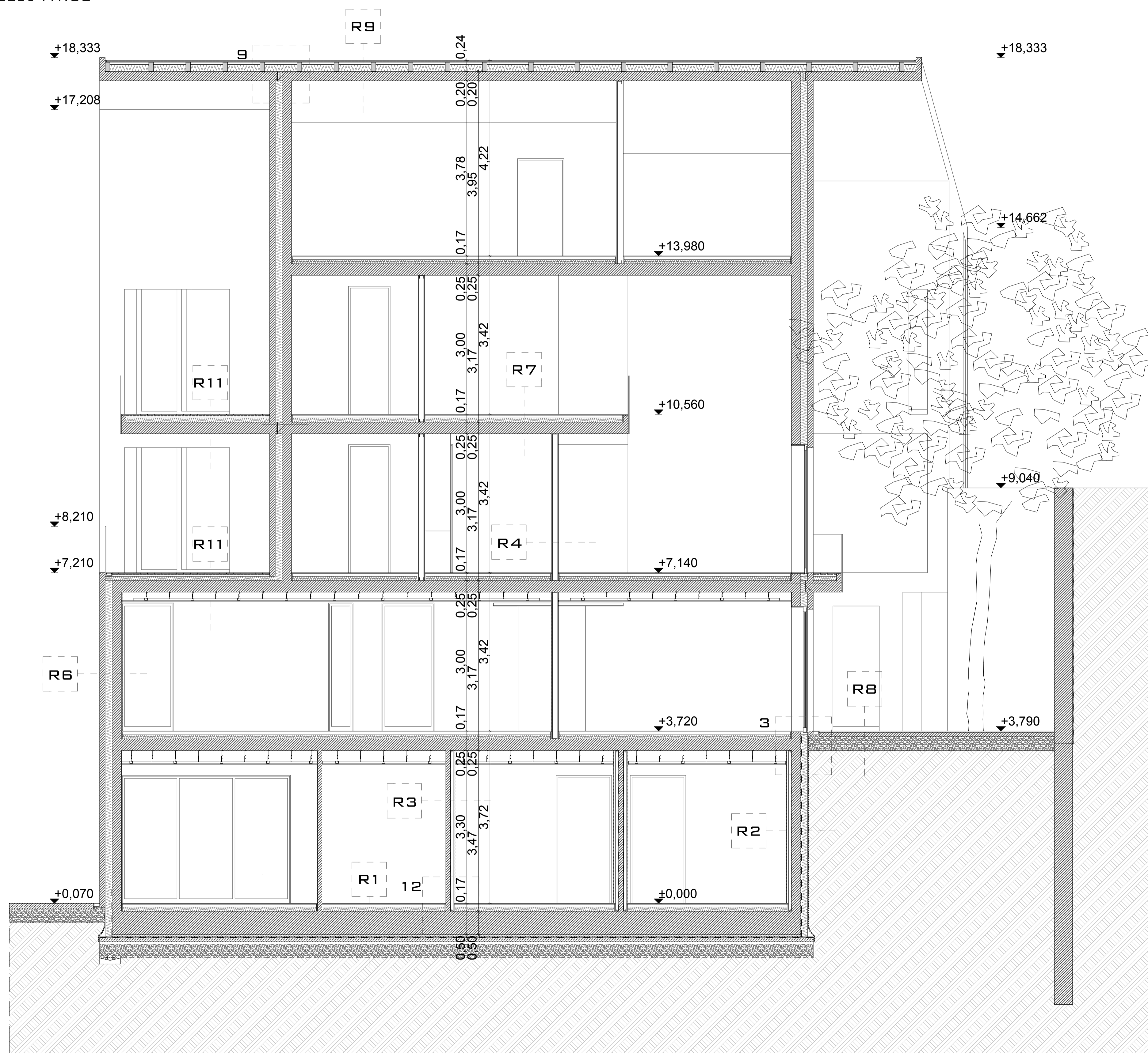
B-B metszet M1:50
