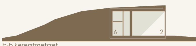
b-b keresztmetszet
