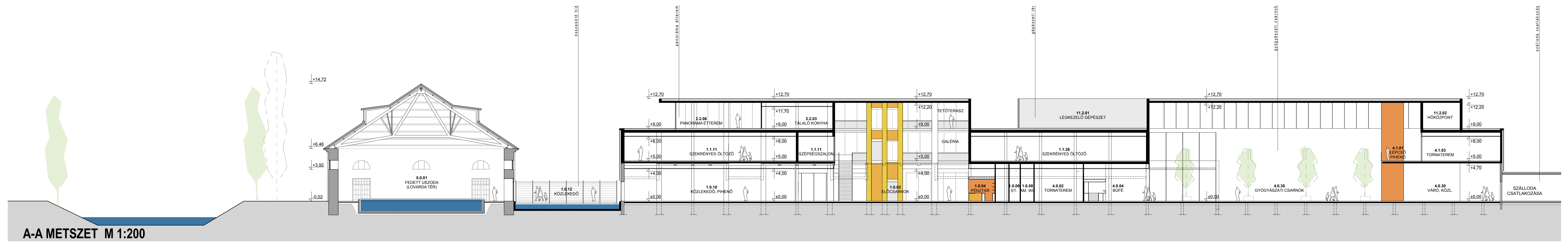
B-B METSZET M 1:200
