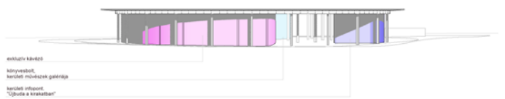
HOMLOKZAT (A-A METSZET) A TELJESEN KINYITOTT PAVILONOK ESETÉN M 1:200
