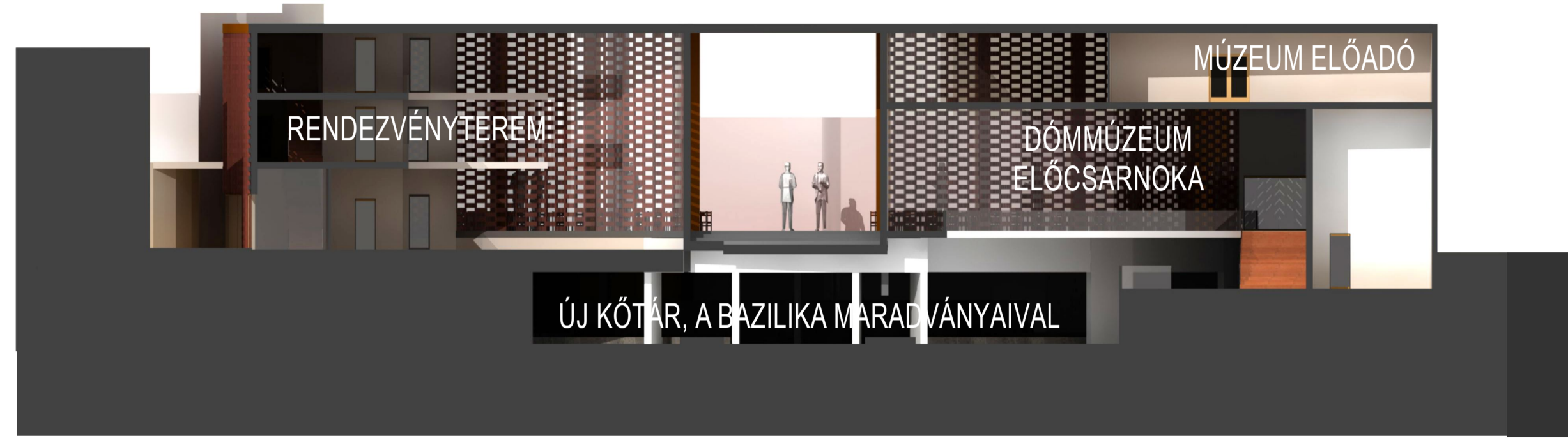
KERESZTMETSZET A MÚZEUMON ÉS A RENDEZVÉNYTERMEN KERESZTÜL
