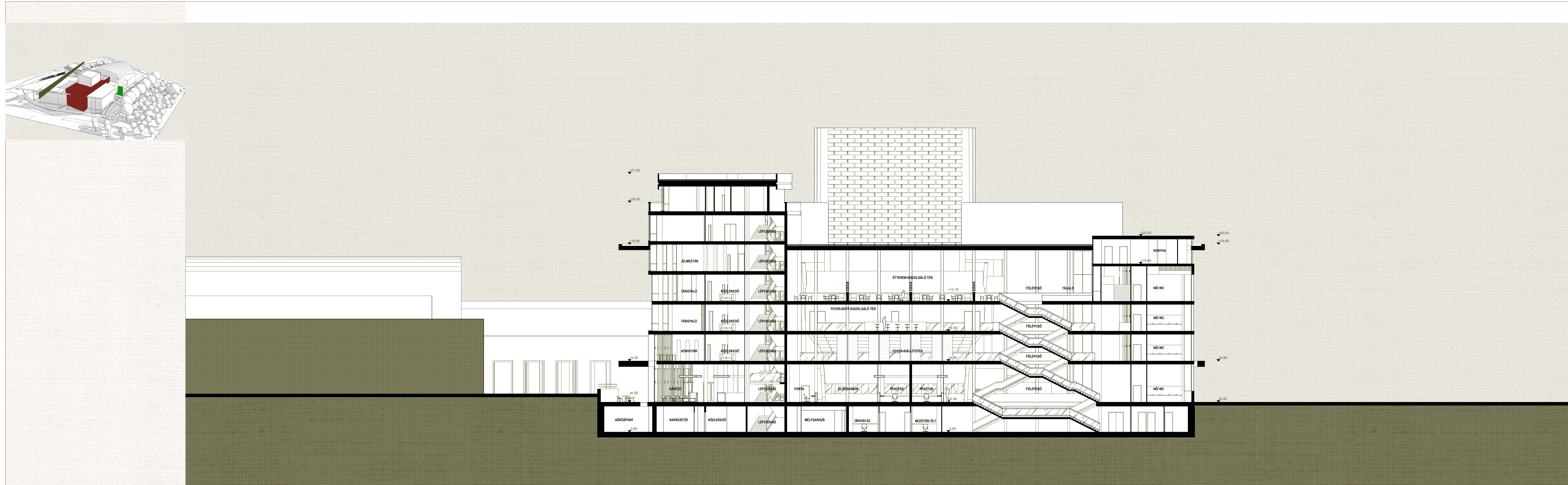
FŐLÉPCSŐ METSZET
