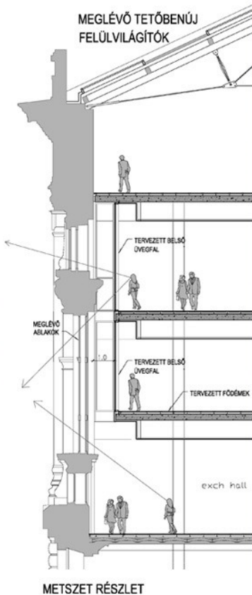
METSZET A VOLT KERESKEDŐCSARNOKON KERESZTÜL
