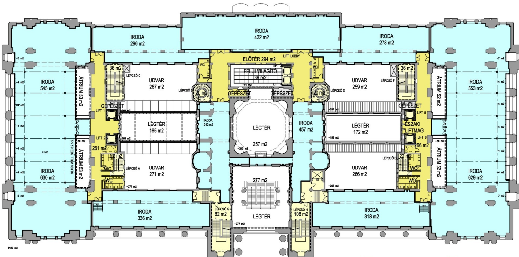
2. EMELET ALAPRAJZA TERVEZETT ÁLLAPOT
