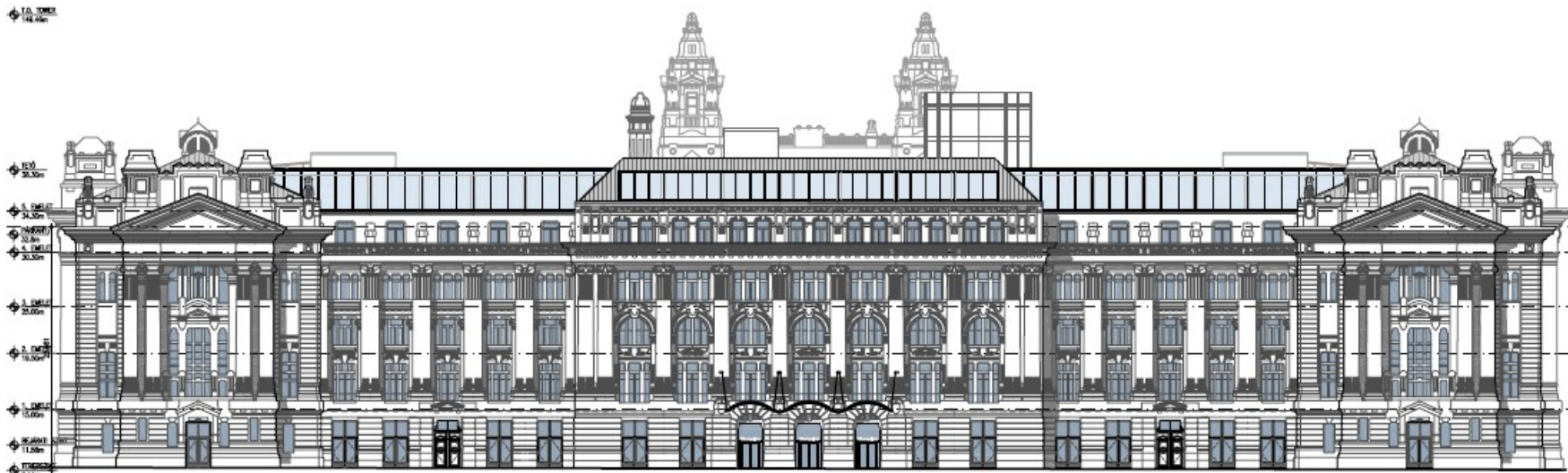
NADOR UTCA (NYUGATI) HOMLOKZAT
