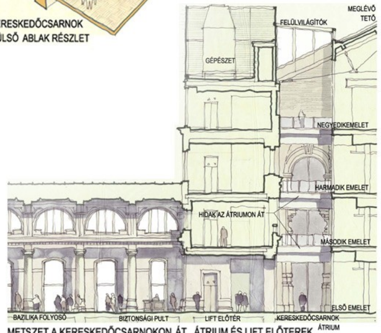
METSZET A KERESKEDŐCSARNOKON ÁT, ÁTRIUM ÉS LIFT ELŐTEREK
