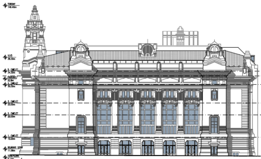
ÉSZAKI (ZOLTAN UTCAI) HOMLOKZAT
