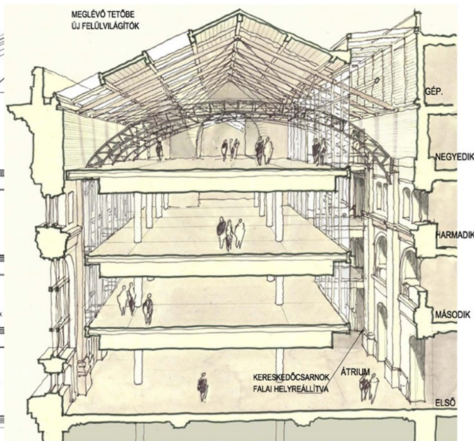
METSZET A VOLT KERESKEDŐCSARNOKON KERESZTÜL
