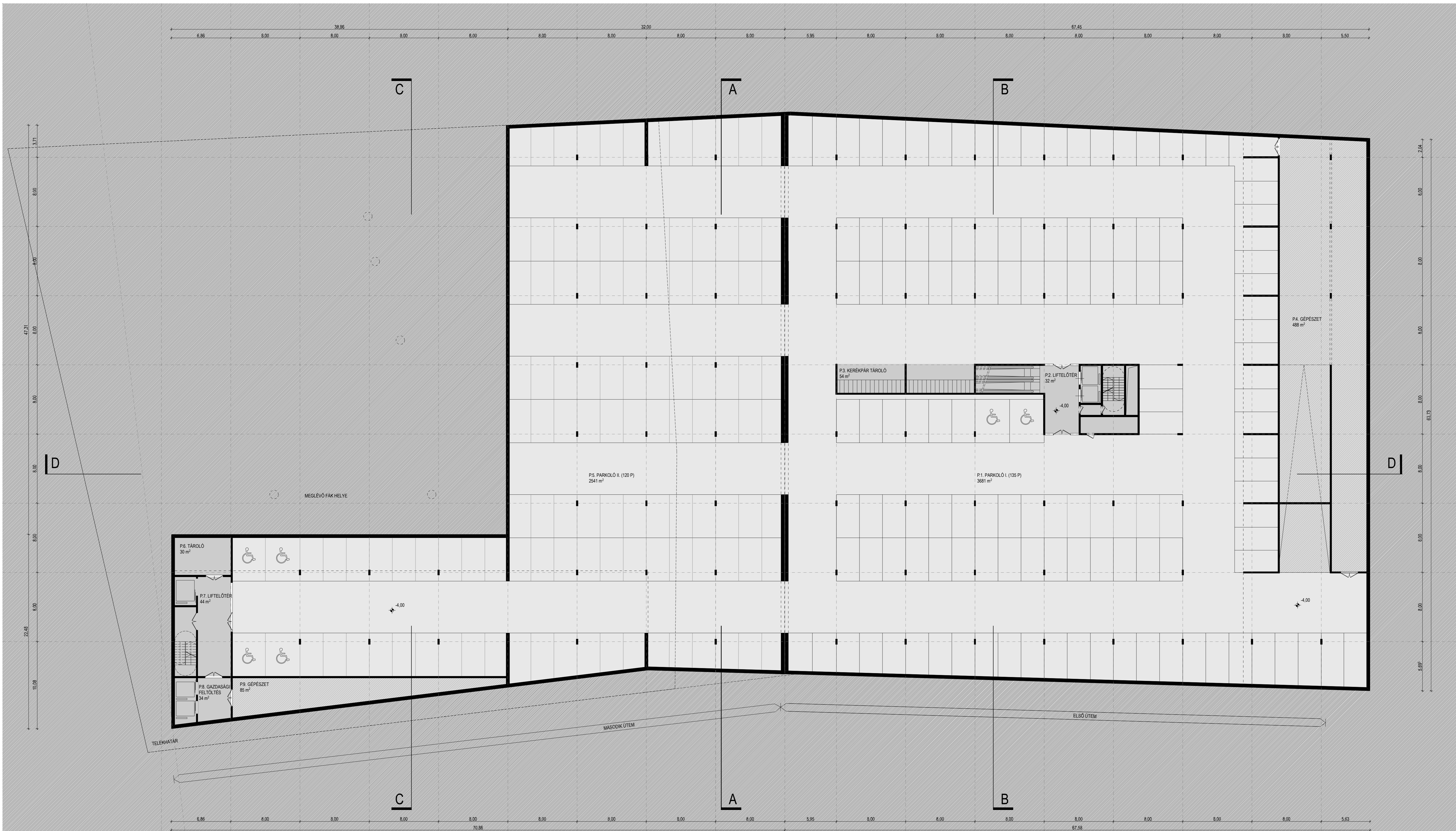
PINCESZINTI ALAPRAJZ M 1:200
