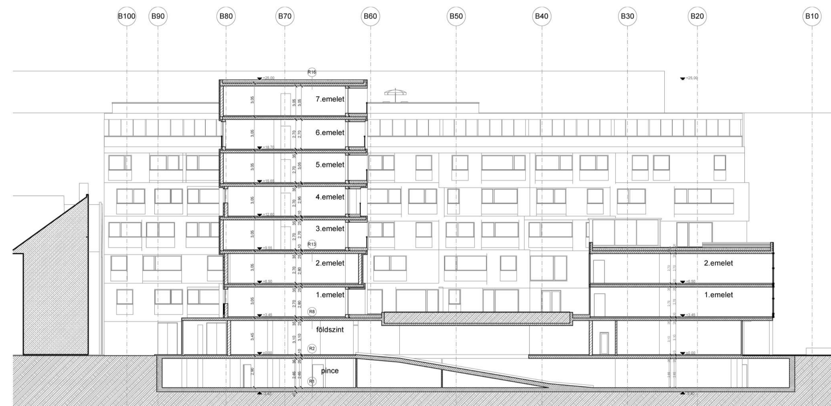
D-D METSZET M 1:200
