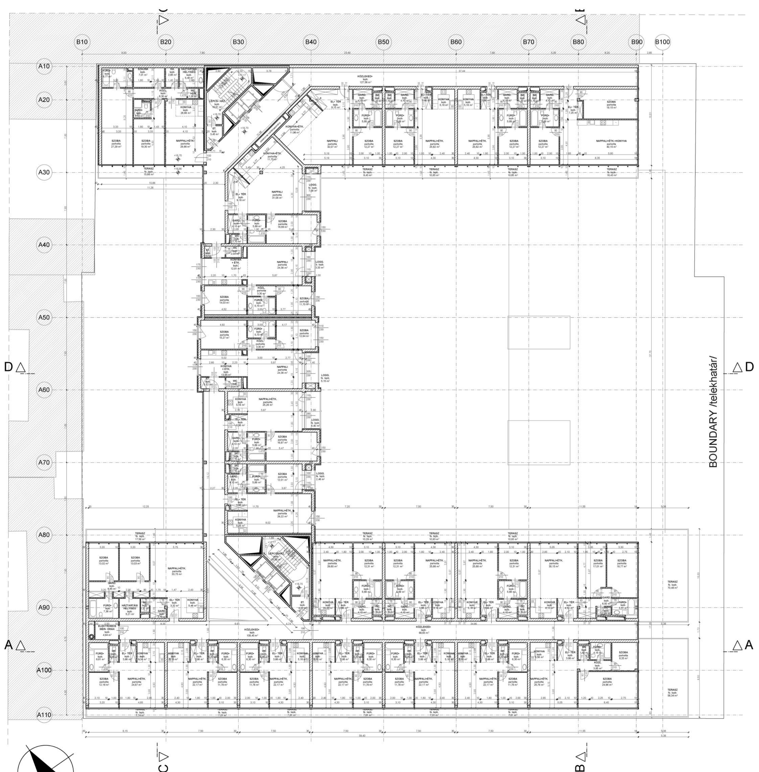
VI. EMELETI ALAPRAJZ M 1:200
