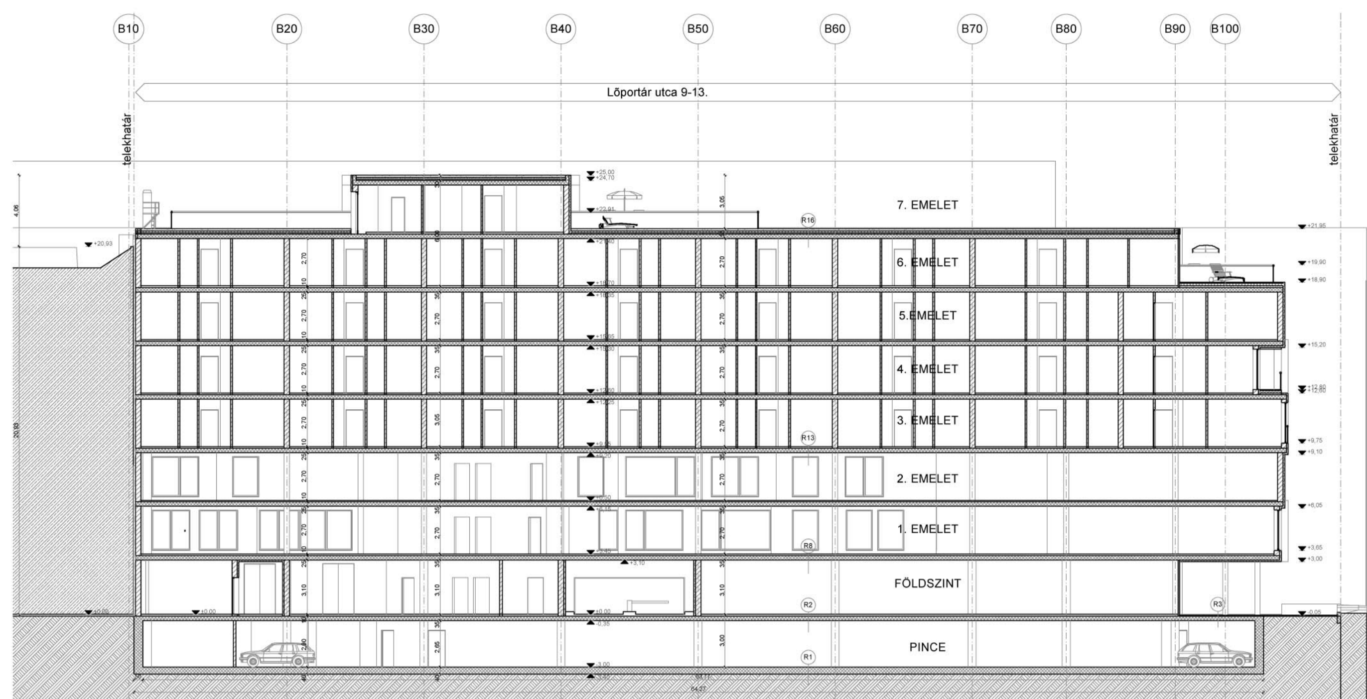
A-A METSZET M 1:200
