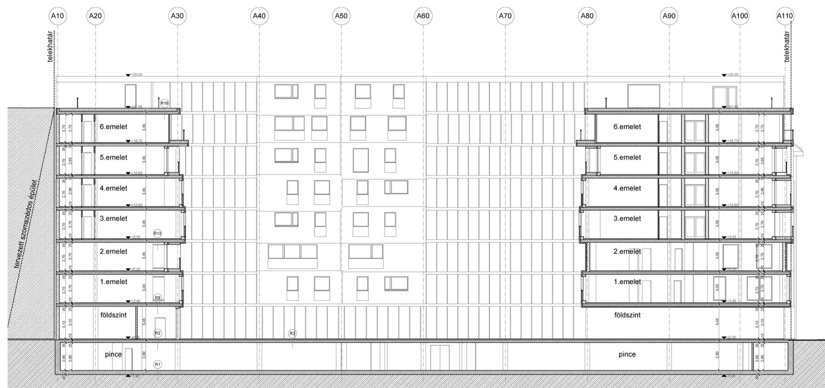
C-C METSZET M 1:200
