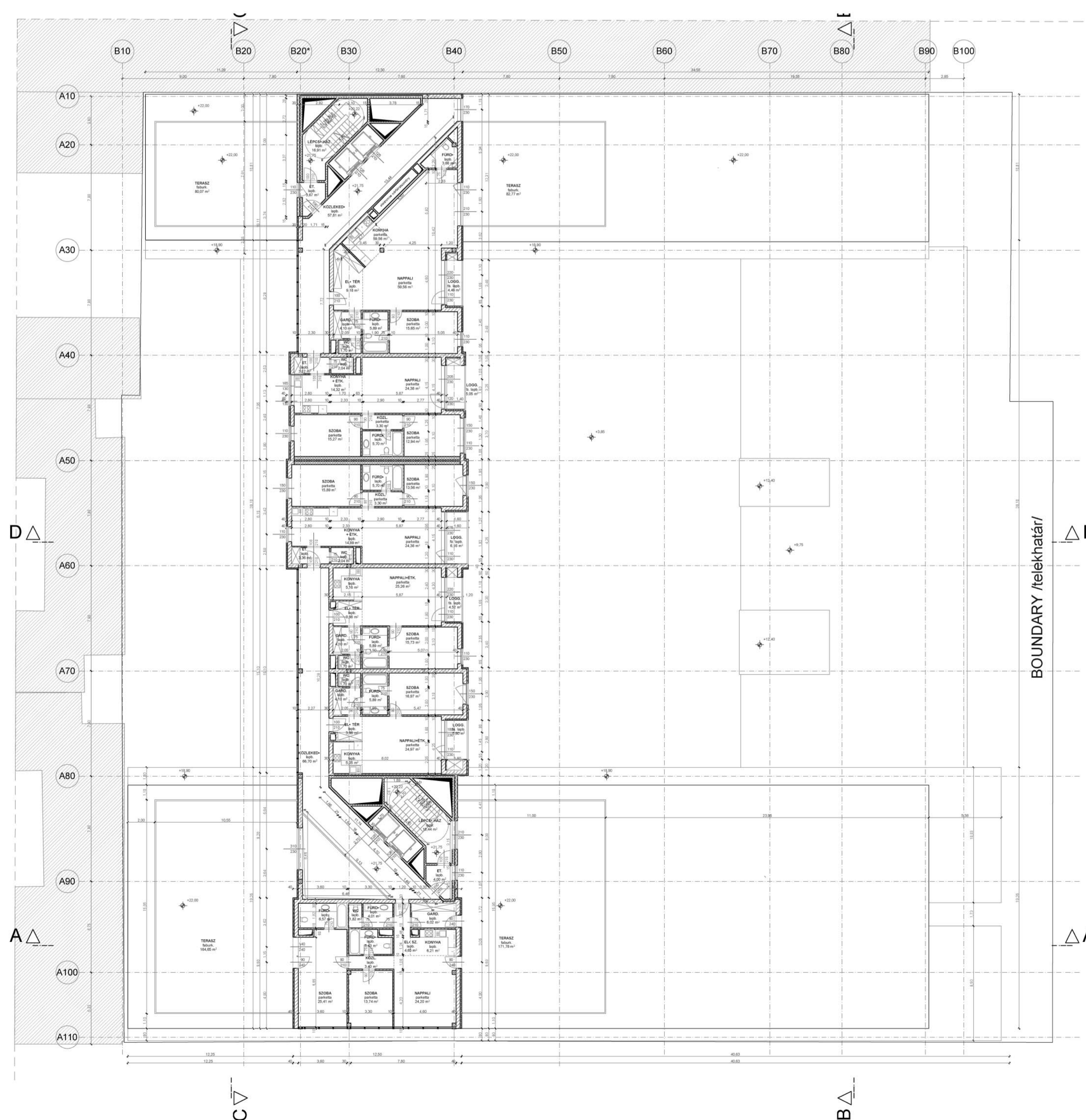
VII. EMELETI ALAPRAJZ M 1:200
