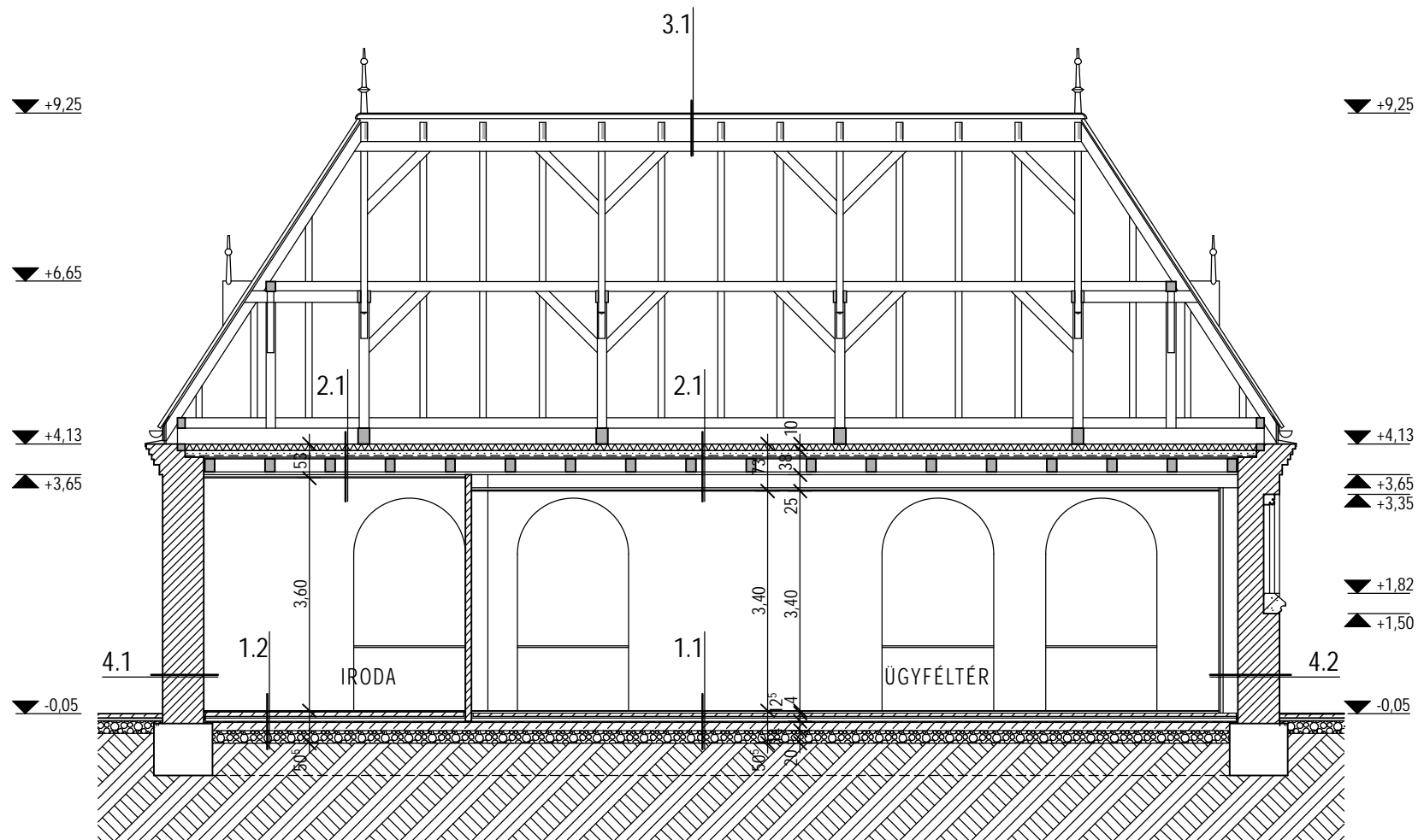
M-M METSZET
