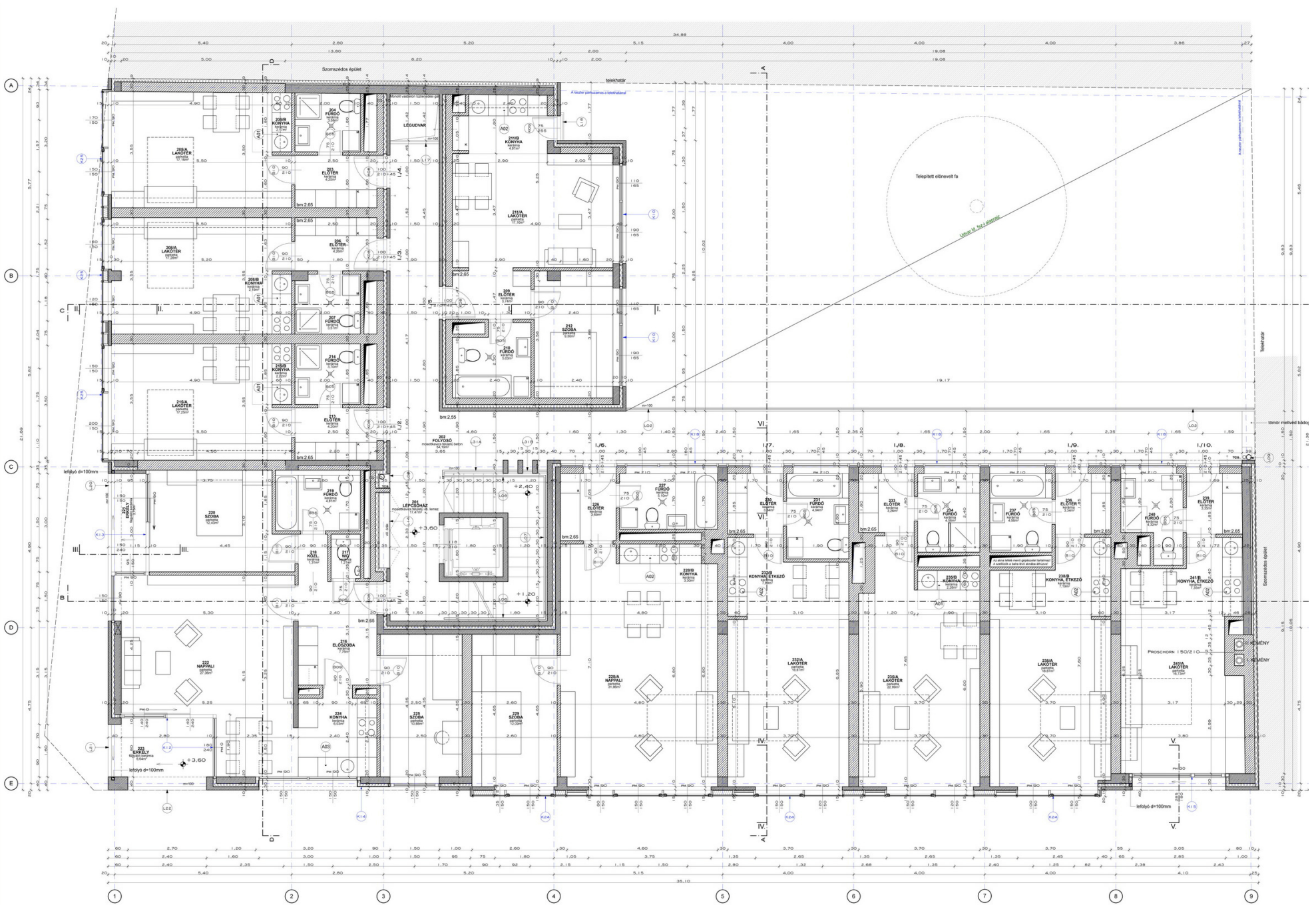
KIVITELI TERV - 1. EMELETI ALAPRAJZ
