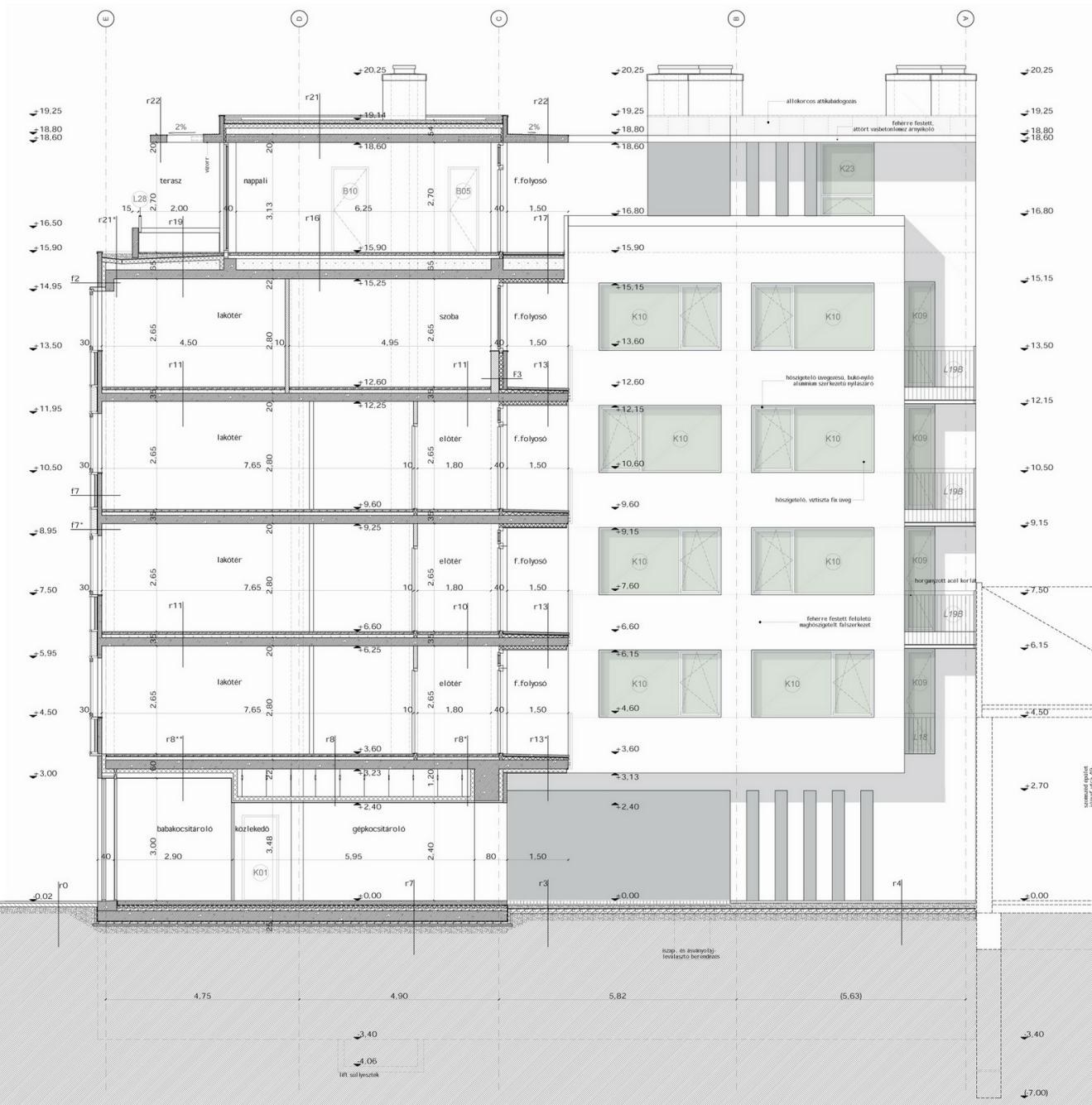
KIVITELI TERV - UDVAR FELŐLI METSZET
