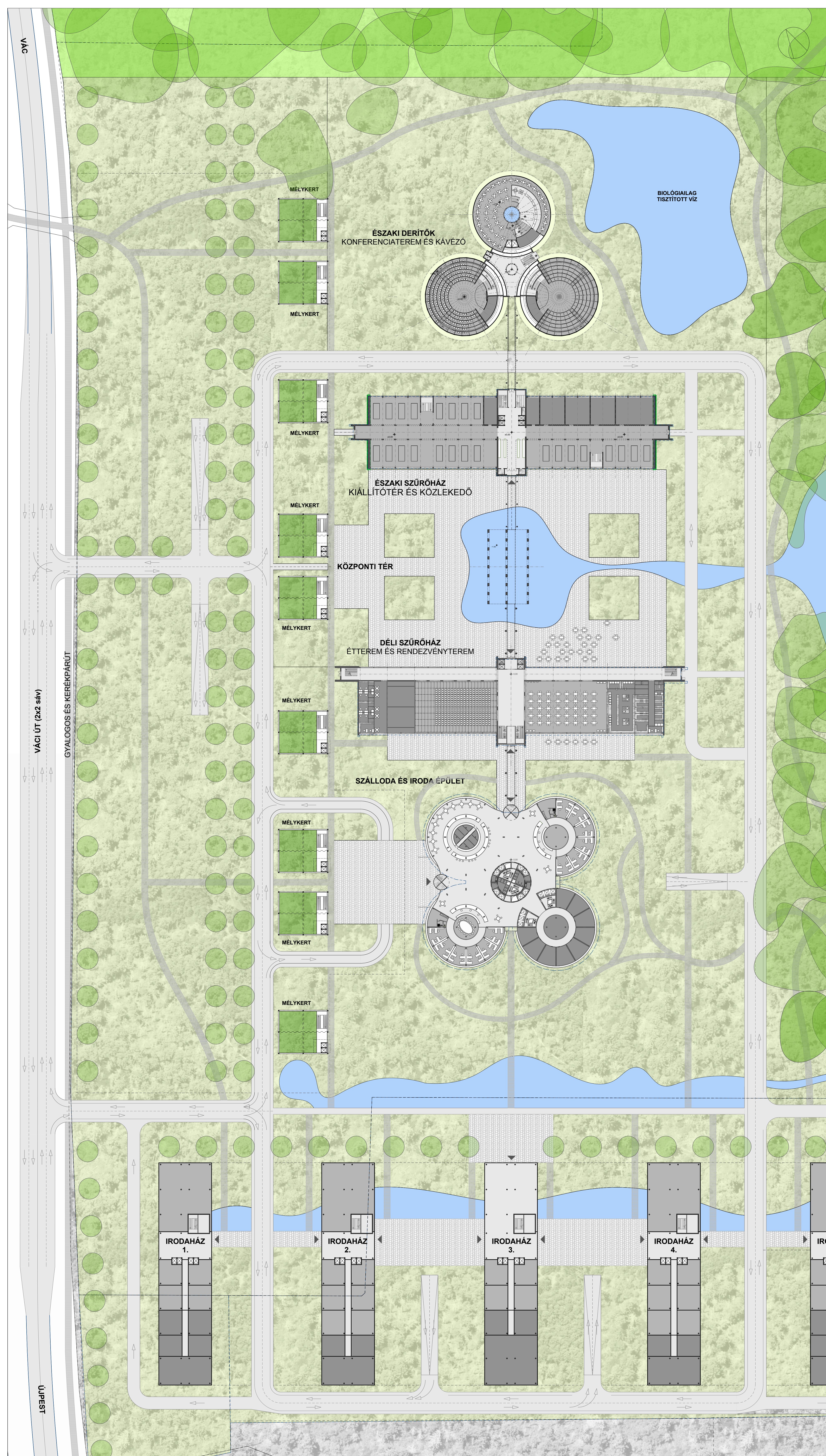
ÚJPEST, VÁCI ÚT 121. NAGYFELSZÍNI VÍZTISZTÍTÓ MŰ HASZNOSÍTÁSÁT CÉLZÓ VÁROSÉPÍTÉSZETI ÖTLETPÁLYÁZAT 2010. VEZÉRSZINTI (FÖLDSZINTI) ALAPRAJZ M=1:500
