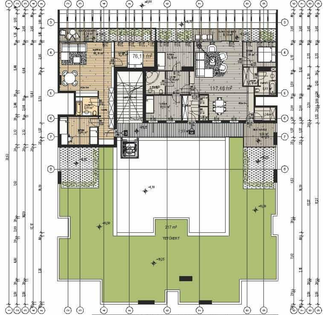
5. EMELETI ALAPRAJZ (második tetőszint)
