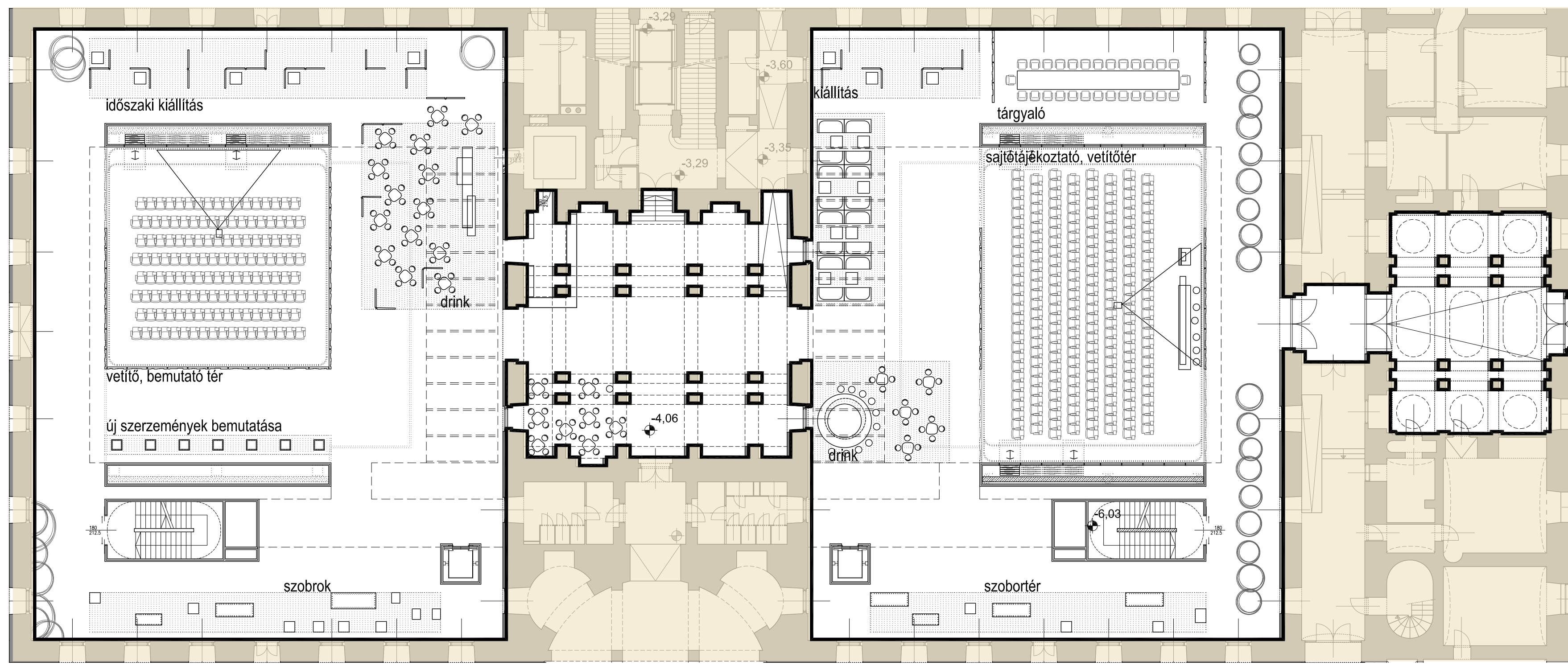
Földszinti alaprajz
