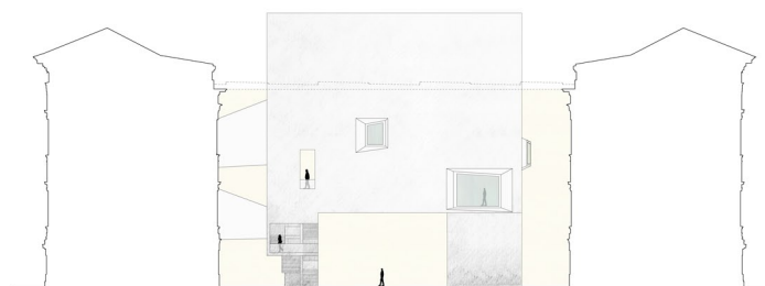
BELSŐ HOMLOKZAT 3 M1:250
