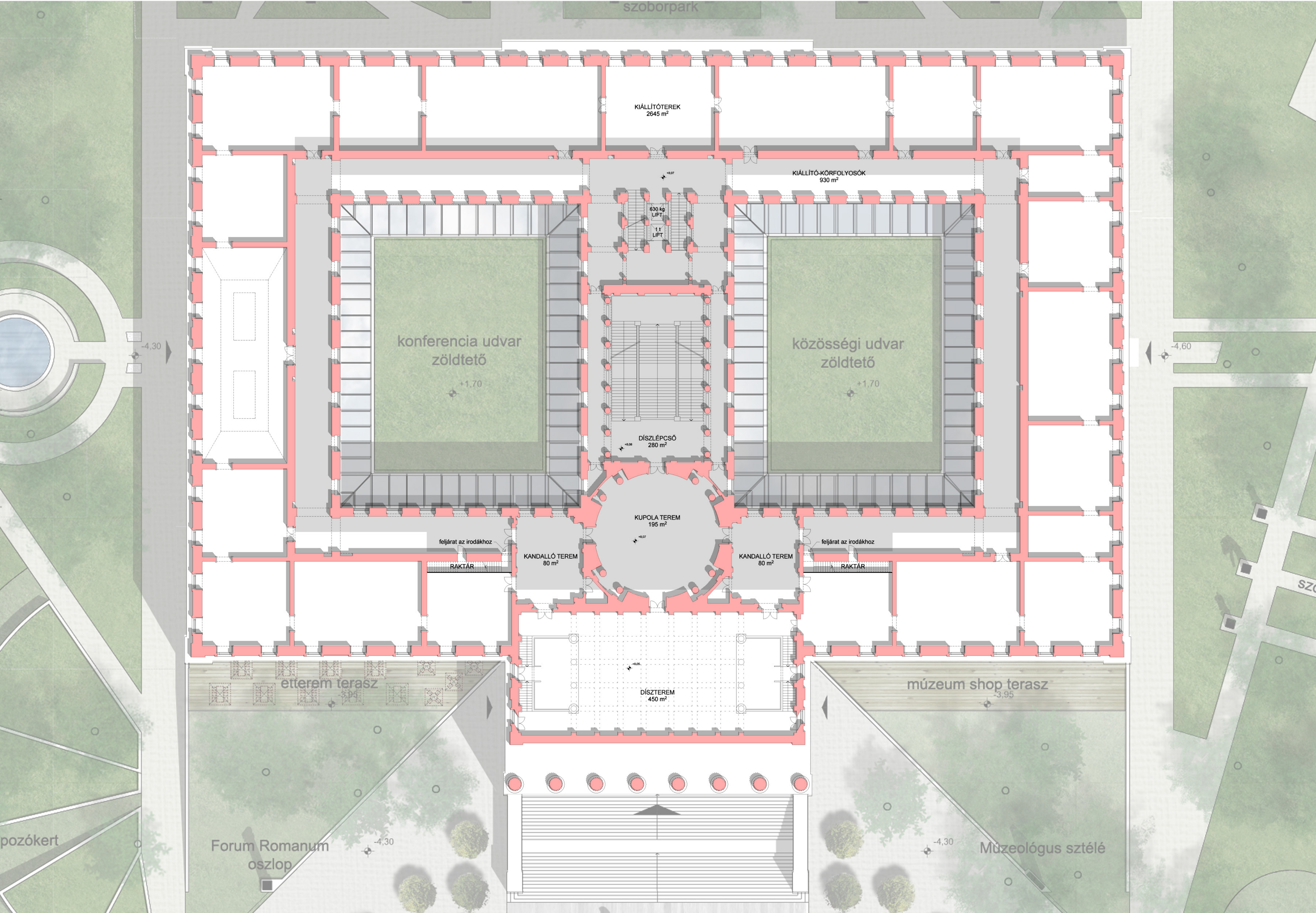
2. emeleti alaprajz - m=1:250
