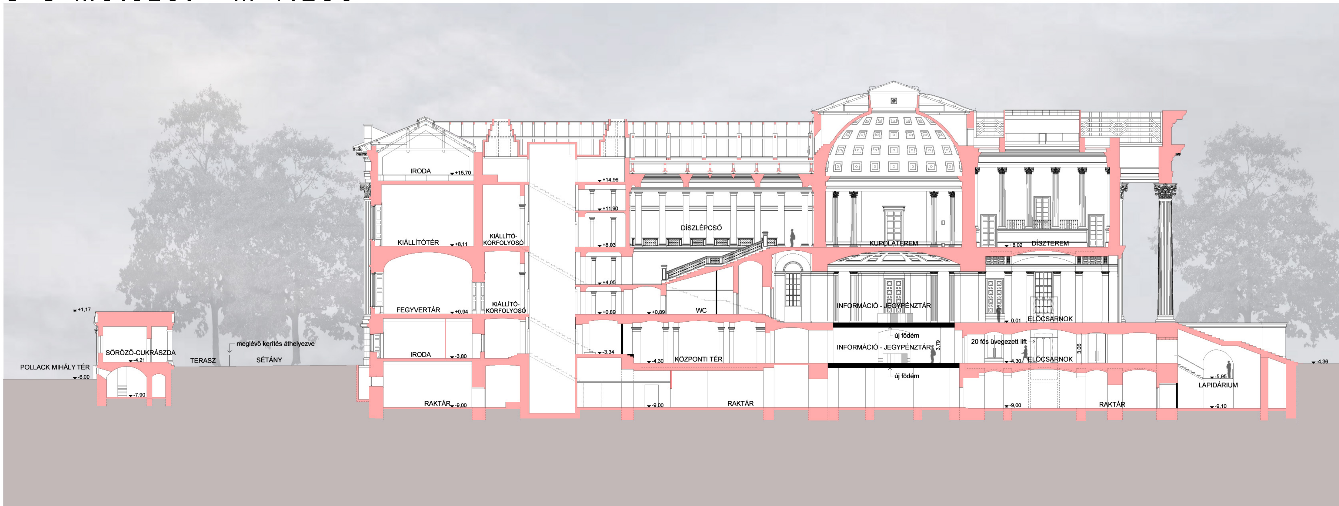
D-D metszet - m 1:250
