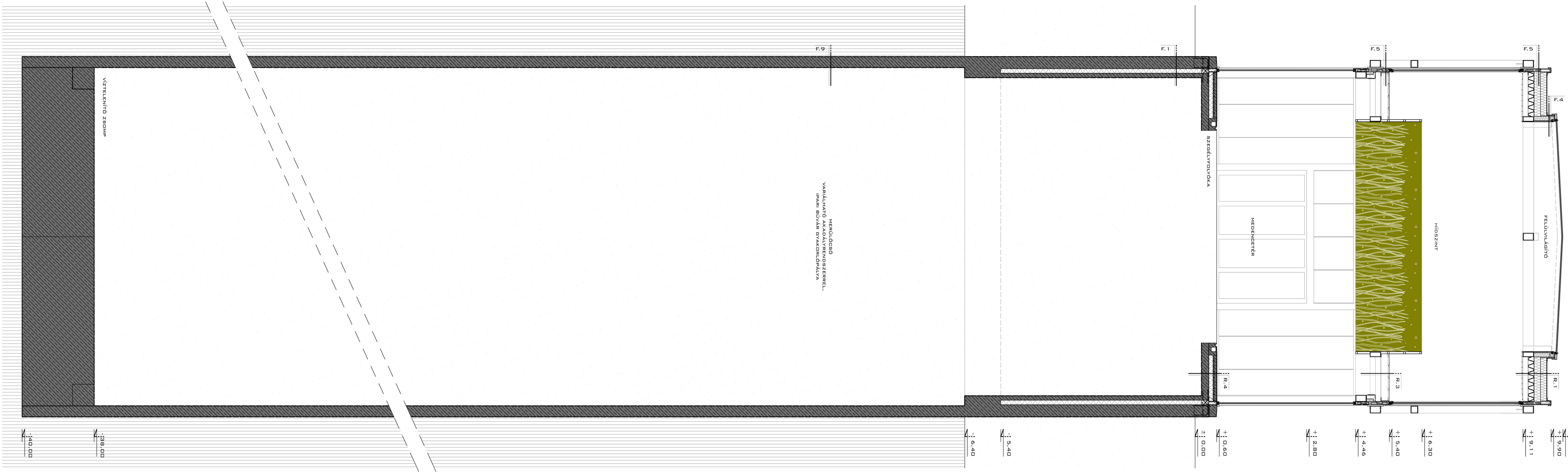
KERESZTMETSZET M 1:50
