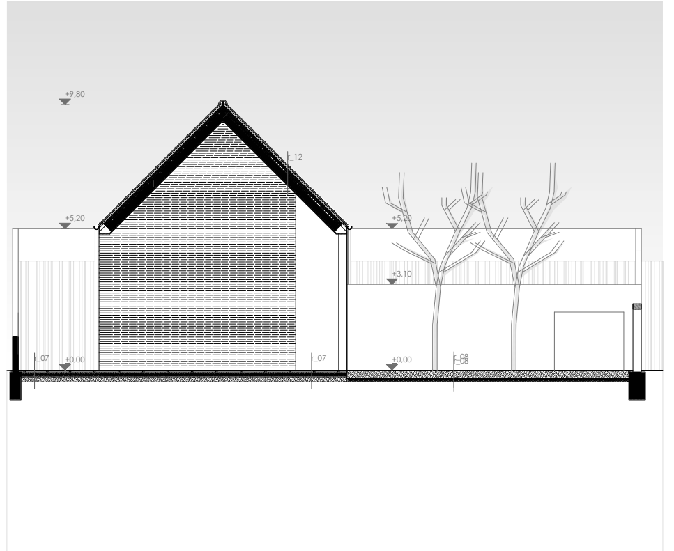
belső északi homlokzat_f-f metszet m_1:100
