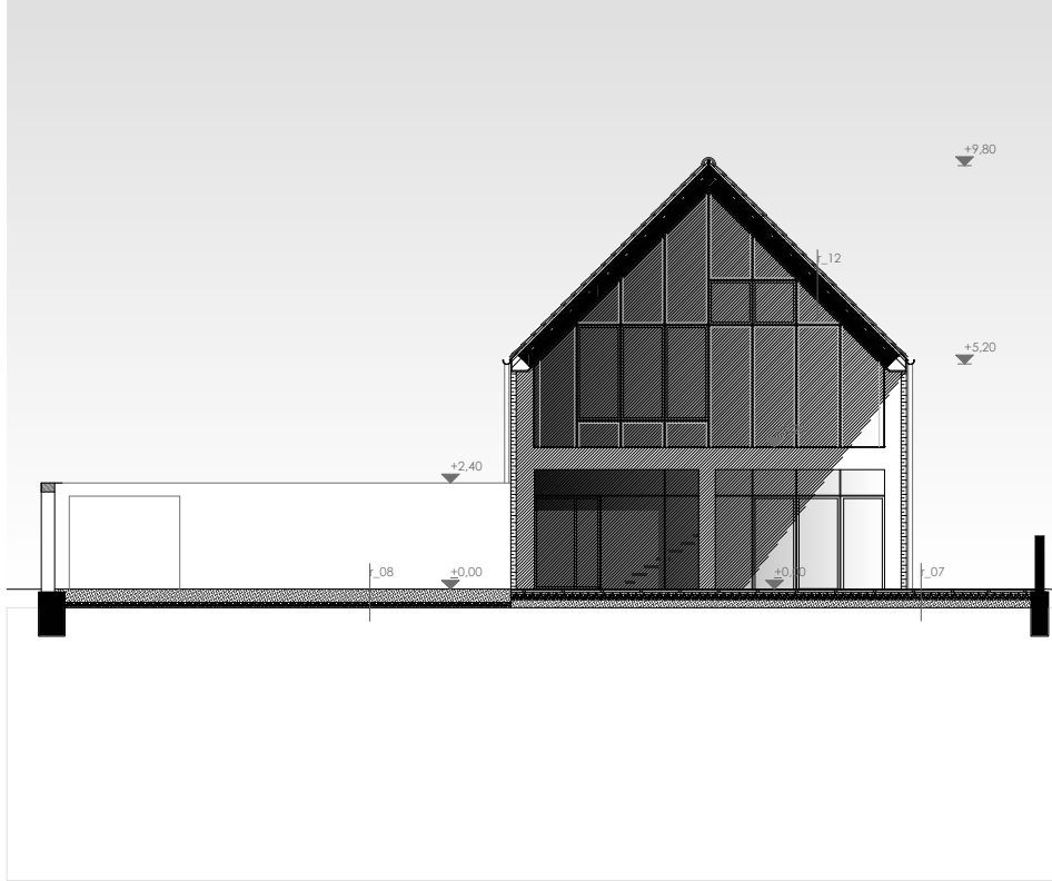
belső déli homlokzat_e-e metszet m_1:100
