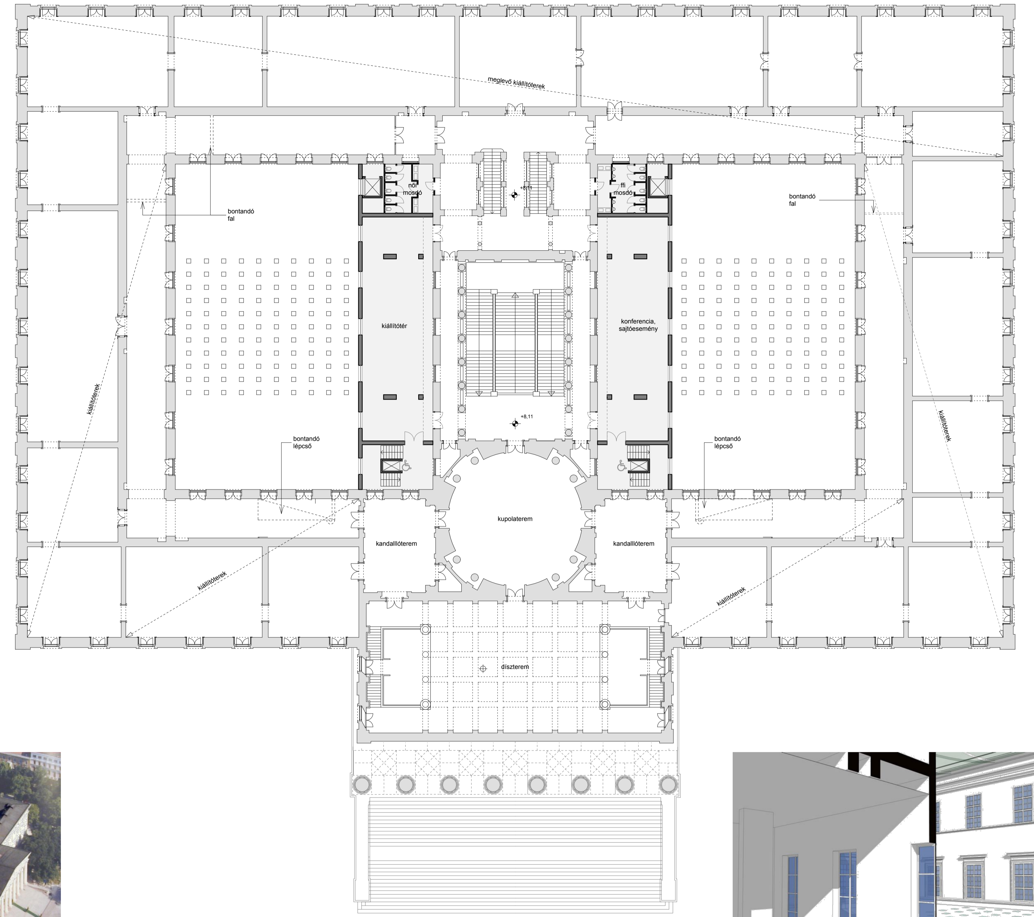
ELSŐ EMELETI ALAPRAJZ (+8,08) M 1:250
