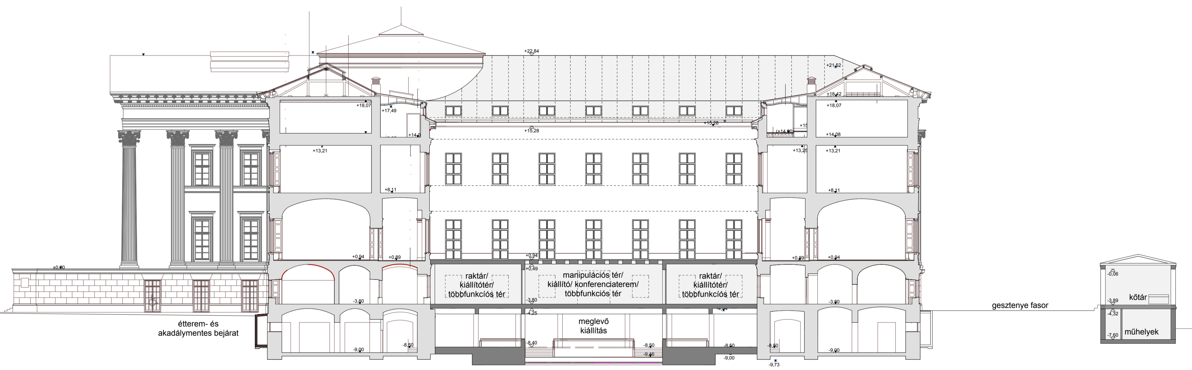
KERESZTMETSZET M 1:250
