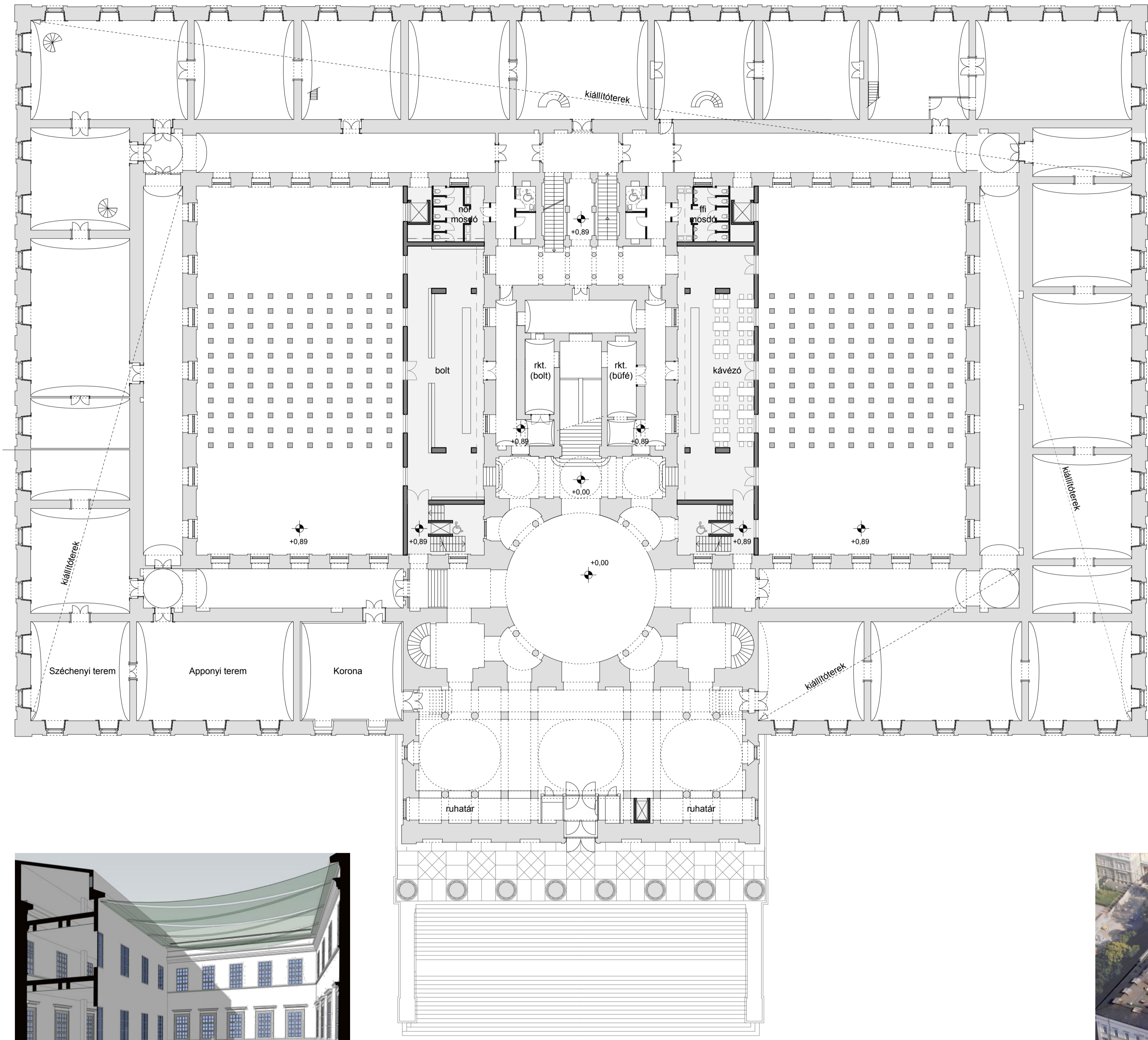
FÖLDSZINTI ALAPRAJZ (0,00) M 1:250
