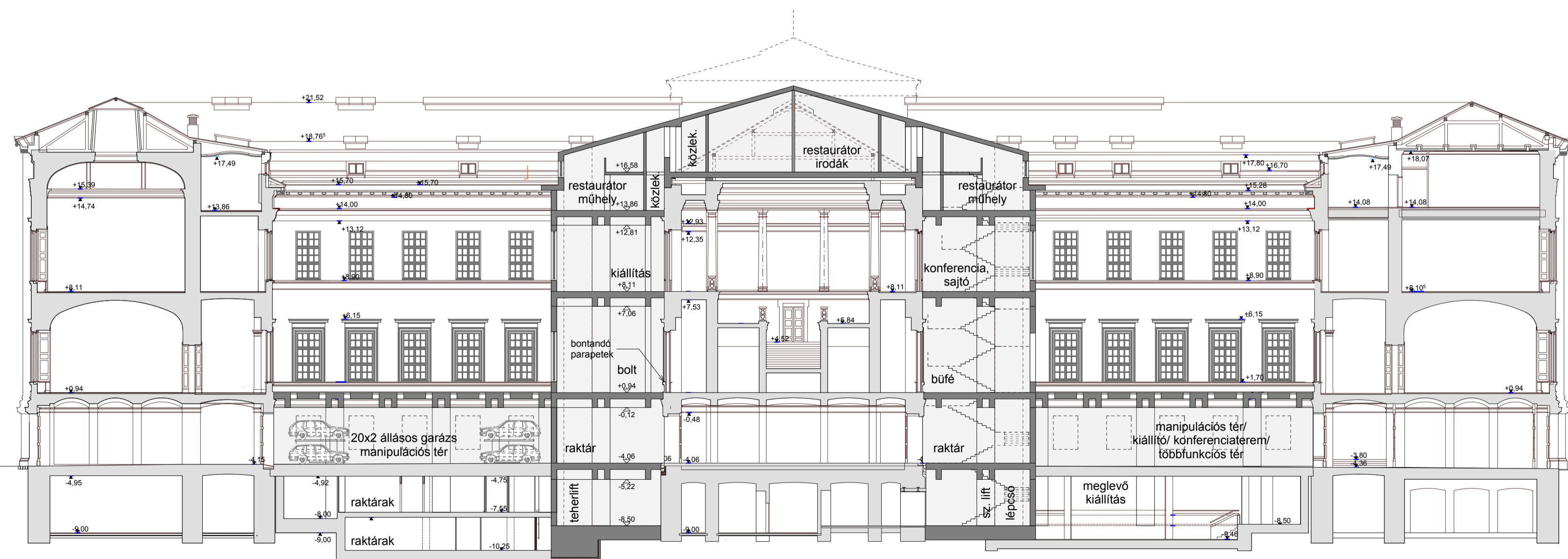
HOSSZMETSZET M 1:250
