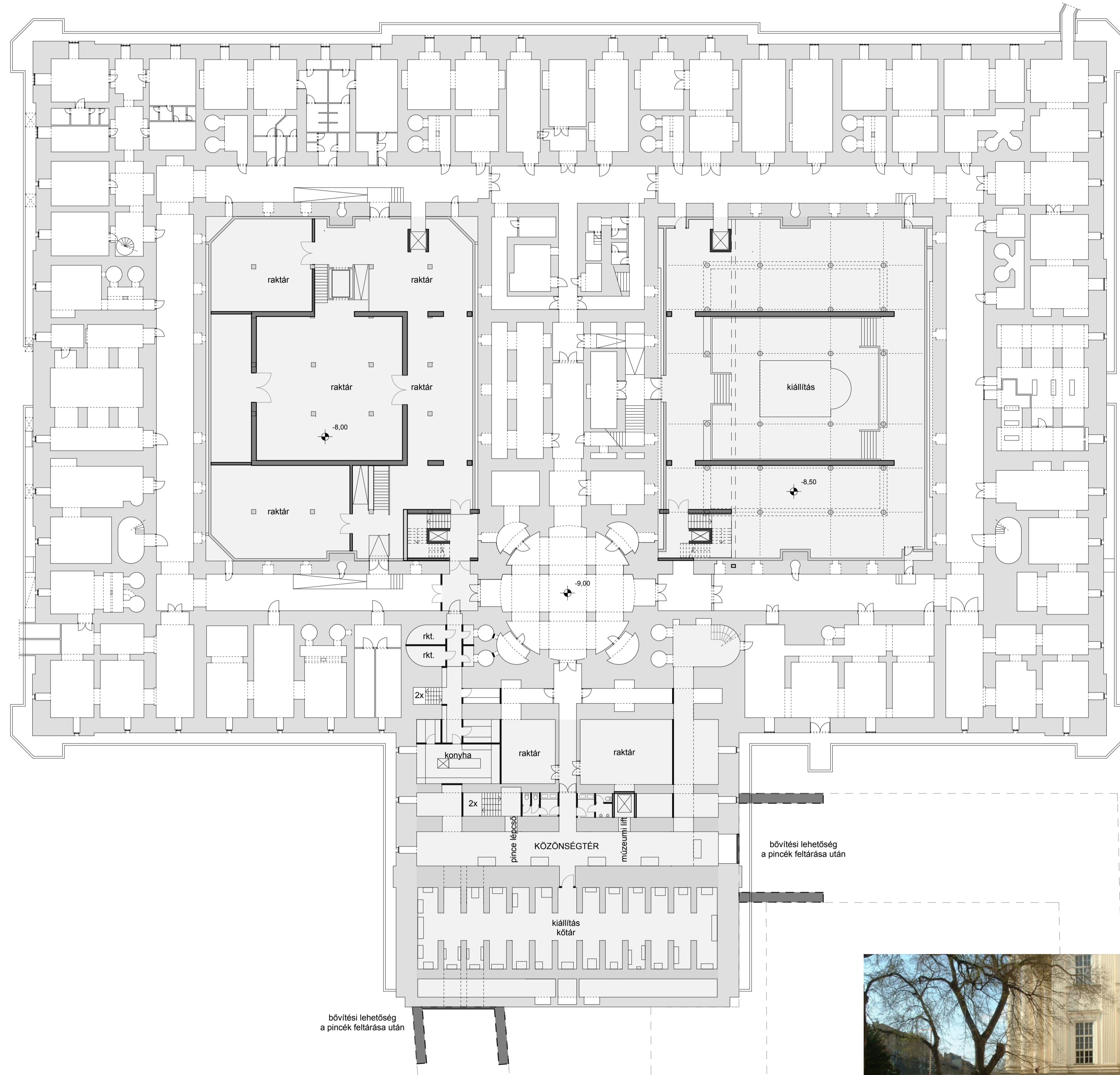
PINCESZINT ALAPRAJZ (-9,00) M 1:250
